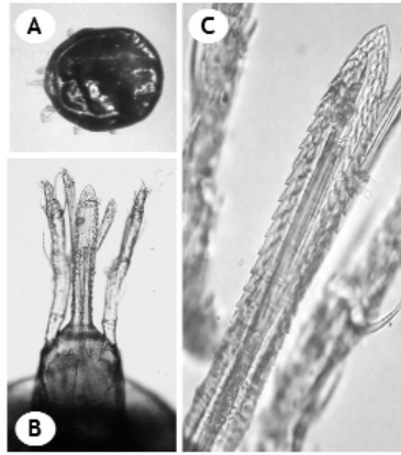
Figura 3. Caracteres diagnósticos de Ornithodoros puertoricensis . A) Vista dorsal de una larva parcialmente alimentada. B) Morfología de la base del capítulo y tamaño de los palpómeros con respecto al hipostoma. C) Hipostoma de una larva con tres hileras de denticulos en la zona apical de la estructura.
