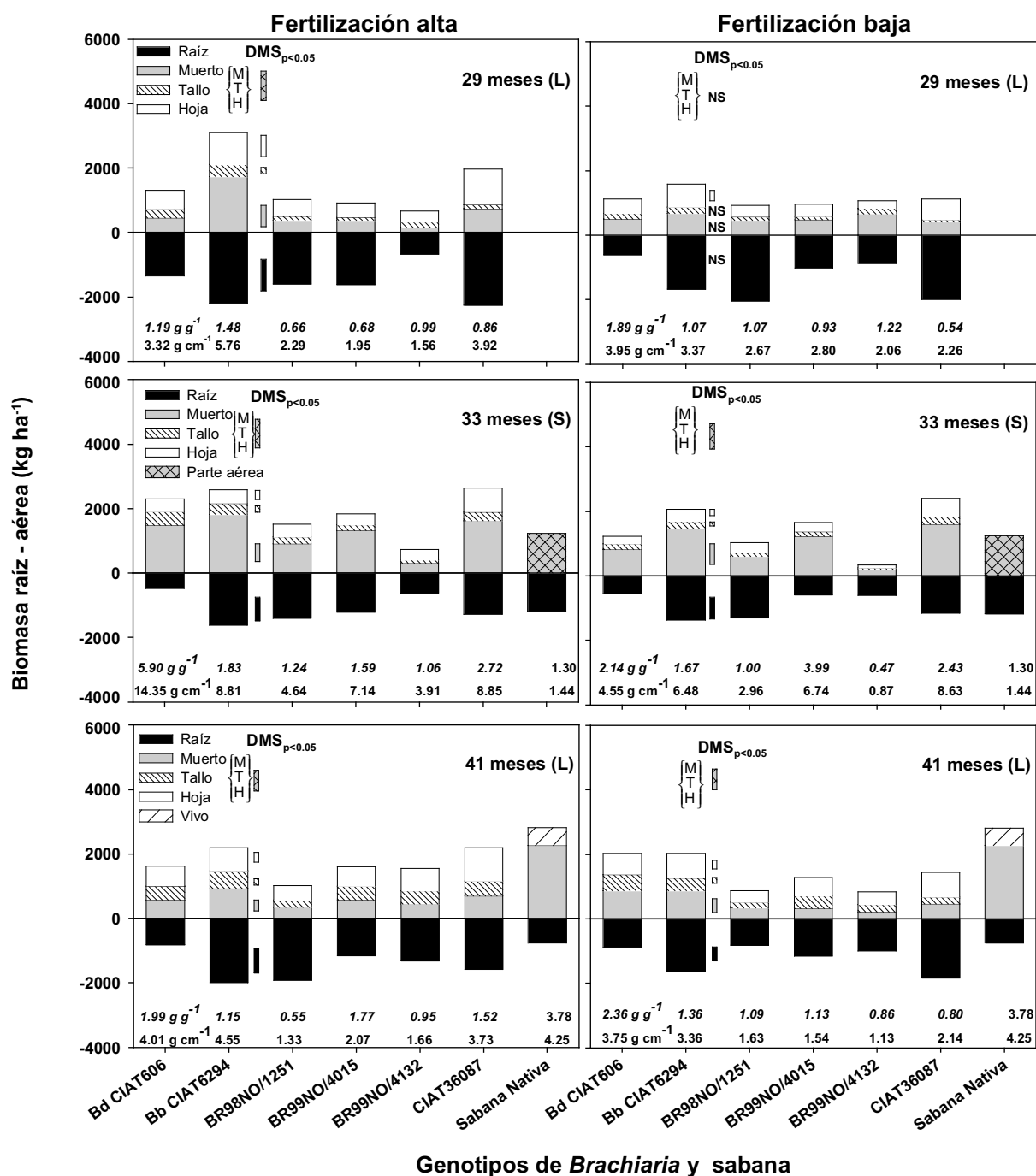
Figura 2. Producción de biomasa de raíces y aérea (kg ha -1 ) en 6 genotipos de Brachiaria , comparados con la sabana, evaluados con alta y baja aplicación de nutrientes a los 29, 33 y 41 meses después de establecidos en un Oxisol de altillanura en Puerto López, Meta (Colombia). Las relaciones producción de biomasa aérea / biomasa de raíz (g g -1 ) y biomasa aérea / longitud de raíz (g cm -1 ) aparecen abajo de las barras correspondientes.
