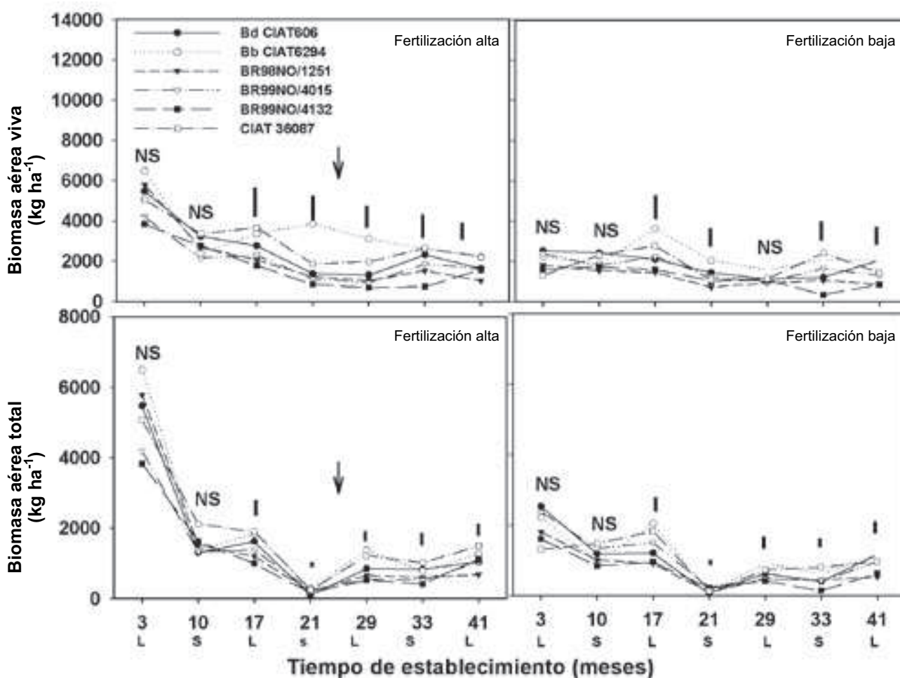
Figura 1. Producción de biomasa aérea ( \text{kg ha}^{-1} ) total (viva + muerta) y viva en 6 genotipos de Brachiaria evaluados durante 3 años (2001 a 2004), al final de las épocas secas (S) y de lluvias (L), en un Oxisol de altillanura en Puerto López, Meta (Colombia), con alta y baja aplicación de nutrientes. Las flechas señalan el momento de adición de la mitad de la dosis alta de nutrientes al tratamiento con altos nutrientes. Las líneas o NS indican los valores de diferencia mínima significativa o diferencia no significativa entre genotipos, respectivamente.
