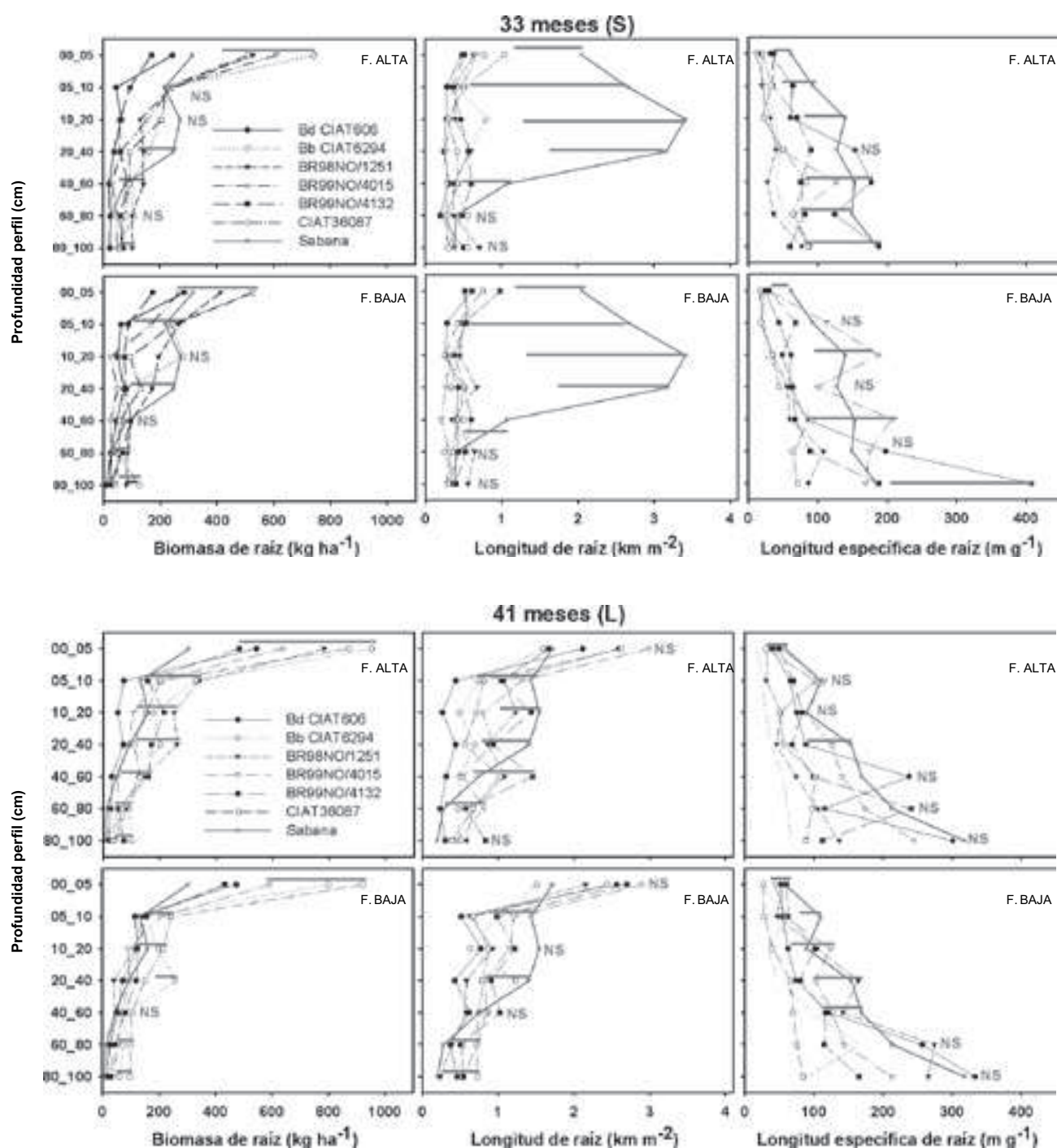
Figura 3. Distribución de la producción de biomasa ( \text{kg ha}^{-1} ), longitud ( \text{km m}^{-2} ) y longitud específica ( \text{m g}^{-1} ) de raíces en 6 genotipos de Brachiaria , comparados con la sabana, 33 (época seca) y 41 (época de lluvias) meses después de establecidos en un Oxisol de altillanura en Puerto López, Meta (Colombia), con alta y baja aplicación de nutrientes. Una línea horizontal o NS en cada profundidad indican, respectivamente, el valor de diferencia mínima significativa o la no diferencia con una probabilidad del 95%.
