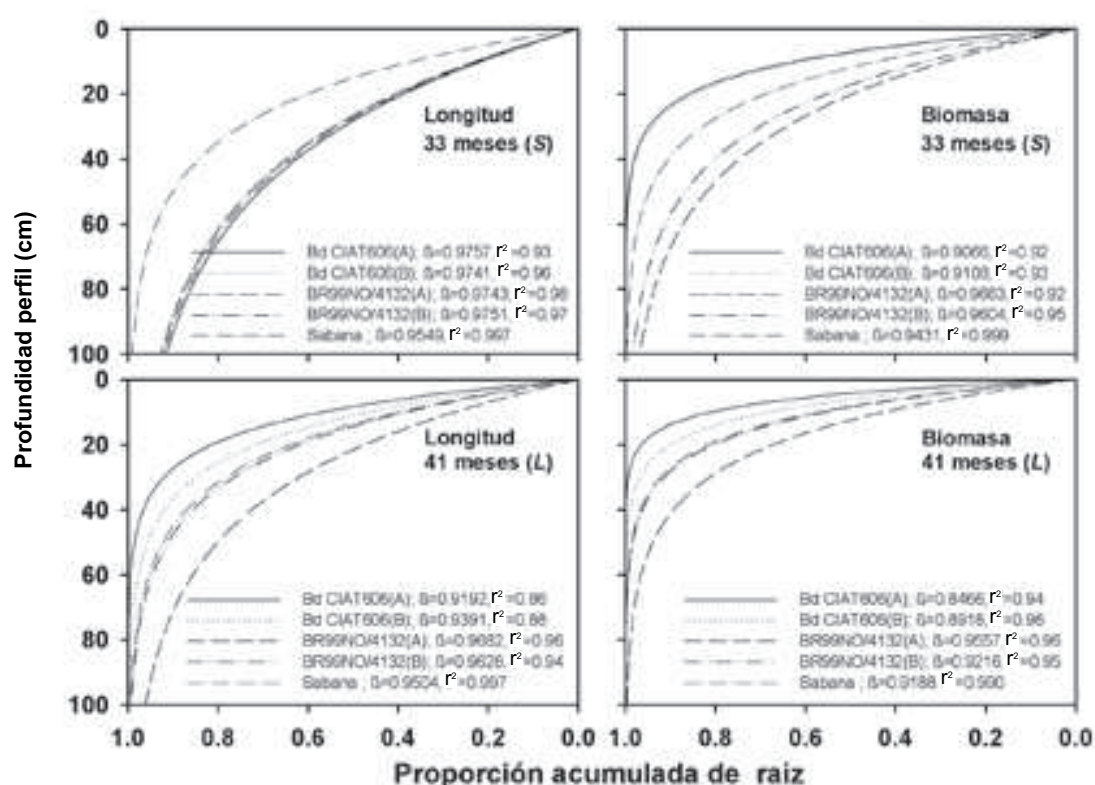
Figura 4. Índice de distribución vertical de raíces, \beta , para la producción de biomasa ( \text{kg ha}^{-1} ) y longitud ( \text{km m}^{-2} ) de raíces en los primeros 100 cm del perfil de suelo de la sabana nativa comparada con 2 genotipos de Brachiaria evaluados a los 33 (época seca - S) y 41 (época lluviosa - L) meses después de establecidos con alta y baja aplicación de nutrientes en un Oxisol de altillanura en Puerto López, Meta (Colombia).
