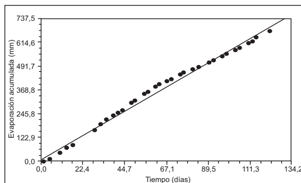
Figura 3. Evaporación acumulada durante el ciclo de cultivo del pimentón Capsicum annuum en el Centro Experimental-CEUNP. Candelaria. 2002
