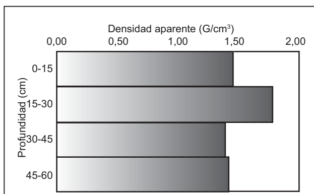
Figura 1. Densidad aparente para cada capa del suelo del Centro Experimental, CEUNP.
