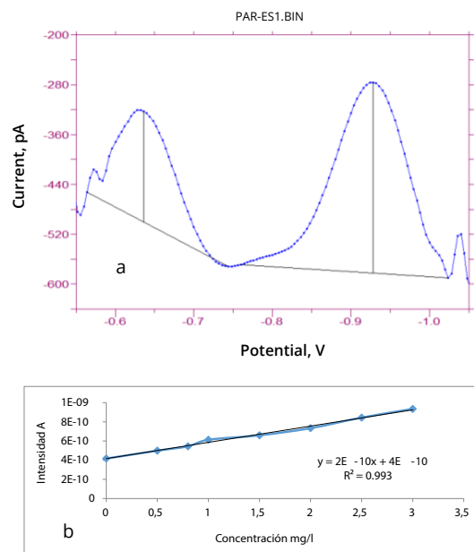
Figura 2. Voltograma de Paraquat por OSWV (a) y curva de calibración (b).
