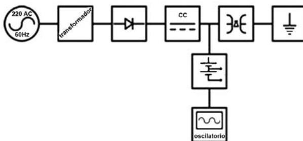
Figura 2. Sistema de generación del campo eléctrico DC compuesto por una fuente de poder, un transformador, un diodo rectificador, un par de electrodos, un divisor de voltaje, un polo a tierra y un osciloscopio
