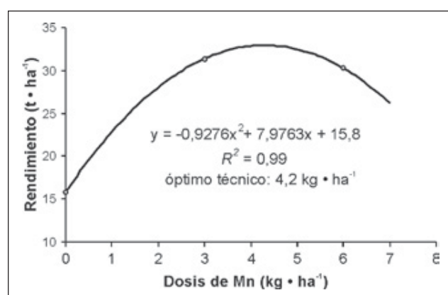
Figura 4. Modelo respuesta del rendimiento de papa ‘Parda Pastusa’ a la aplicación de Mn en un Typic Hapludands del altiplano Cundiboyacense.
