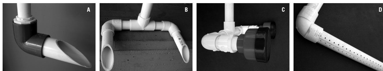
FIGURA 3. Boquillas evaluadas: descarga libre (A), cacho doble (B), poma 400 y 1.000 (C) y flauta (D).
