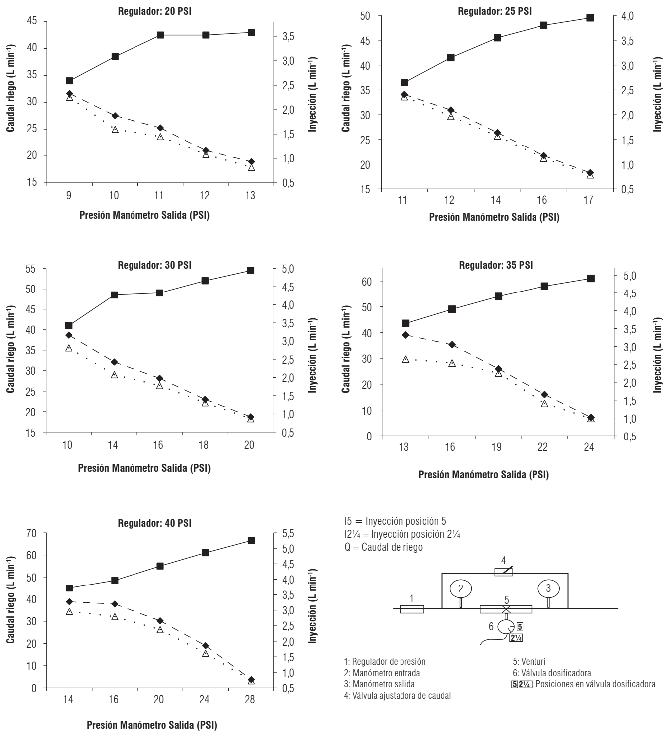
FIGURA 11. Nomograma CG5. Diámetro del venturi (DV) 2,54 cm; diámetro de la manguera (DM) 2,54 cm; largo de la manguera (LM) 75 m. ---◆--- I15, ---△--- I2 1/4, —■— Q riego.
