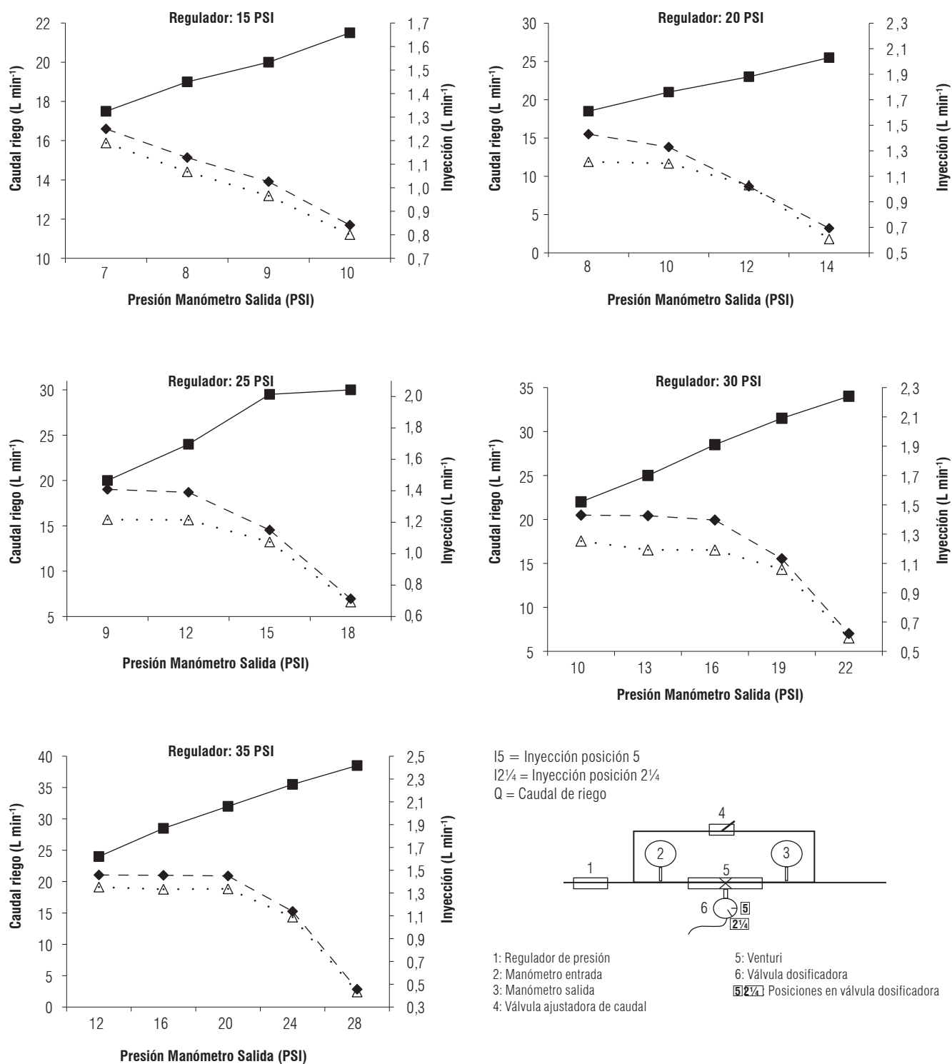
FIGURA 10. Nomograma CG4. Diámetro del venturi (DV) 1,9 cm; diámetro de la manguera (DM) 1,9 cm; largo de la manguera (LM) 50 m. ---◆--- I15, ---△--- I2¼, —■— Q riego.
