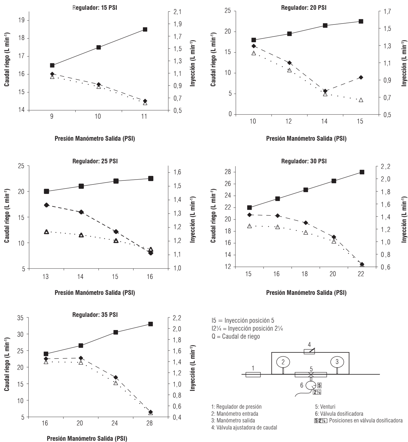
FIGURA 9. Nomograma CG 3. Diámetro del venturi (DV) 1,9 cm; diámetro de la manguera (DM) 1,9 cm; largo de manguera (LM) 75 m. ---◆--- I15, ...△... I2 1/4, —■— Q riego.
