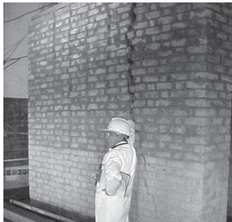
Figura 14: Montaje y mecanismo de falla del primer muro. Grieta vertical dominante debida a tensión en el mortero.
