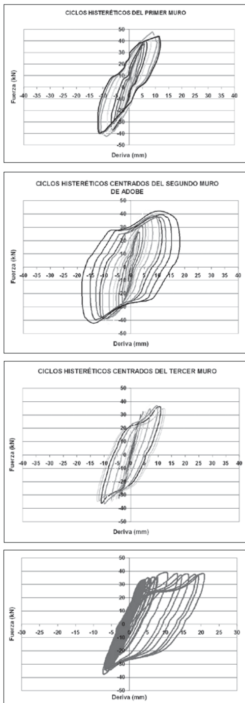
Figuras 17 a 19: Ciclos histeréticos para los muros ensayados.
