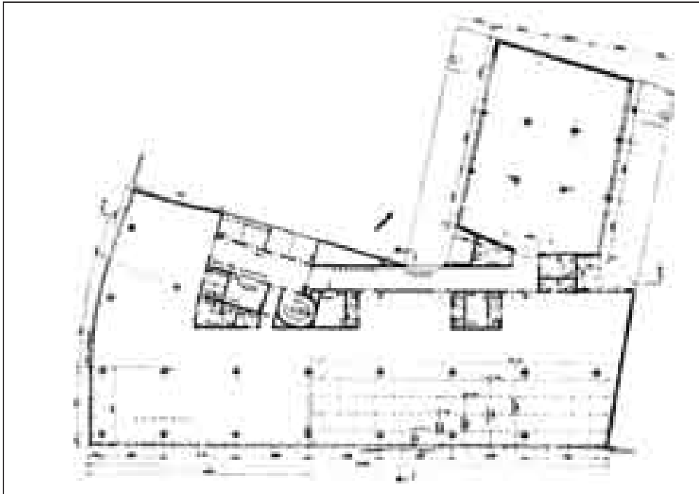
Figura 12: Rino Levi. Banco Paulista do Comércio, São Paulo, 1947. Plano de los pisos superiores.
