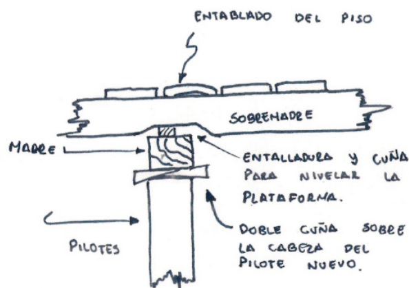
Figura 10: Detalle del remplazo de los pilotes deteriorados y como se adhieren a la estructura existente
