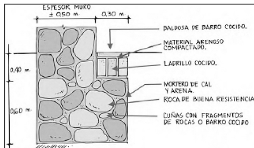
Figuras 25 y 26: Viga de cimentación y sobrecimiento Fuente: AIS (2004, pp. 20 y 22)
