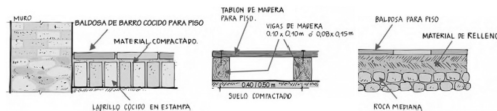
Figura 27: Distintas configuraciones para pisos de construcciones en tapia pisada Fuente: AIS (2004, p. 23)
