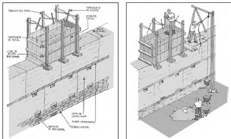
Figuras 28 y 29: Esquema de la construcción de una edificación en tapia pisada
