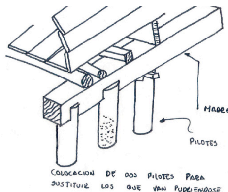
Figura 9: Diagrama de colocación de los pilotes (arriba) y estructura de piso (abajo) Fuente: Modificado de Mallol y De Recasens, 1963
