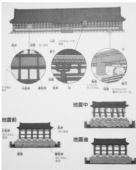
Figura 24: El sistema de protección contra sismos en el Templo de Sanjōsangen- dō en Kioto
