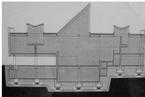
Figuras 35 y 36: Tokio, National Western Art Museum, proyecto de Le Corbusier (1959). Aislamiento en la base para proteger el edificio (1999)
