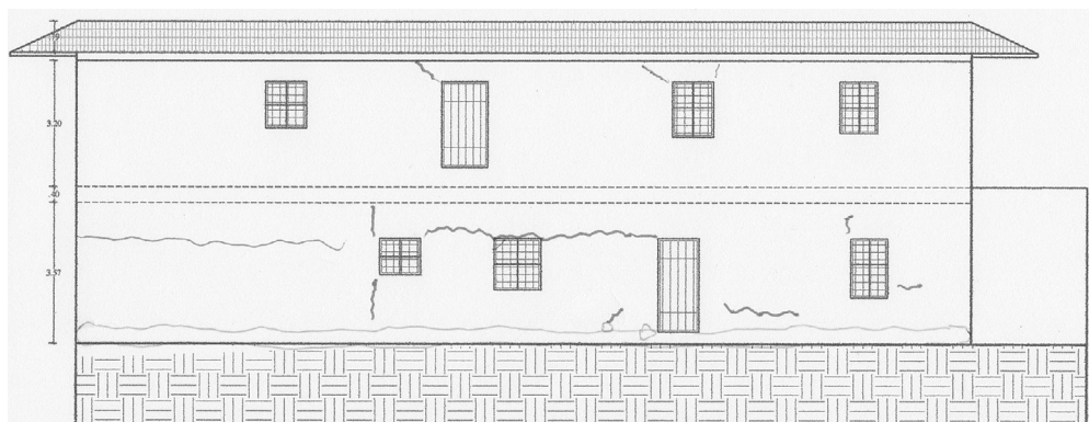
Figura 15: Fisuras en muros de fachada posterior de la casa consistorial de Cogua Fuente: elaboración propia
