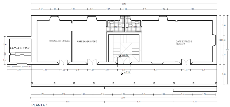
Figura 8: Planta arquitectónica del primer piso de la casa consistorial de Cogua Fuente: elaboración propia
