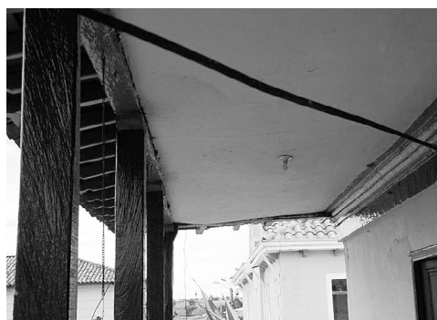
Figura 21: Cielos rasos sobre el sector del corredor del segundo piso, que presenta deformaciones y fisuras Fuente: Archivo de los autores
