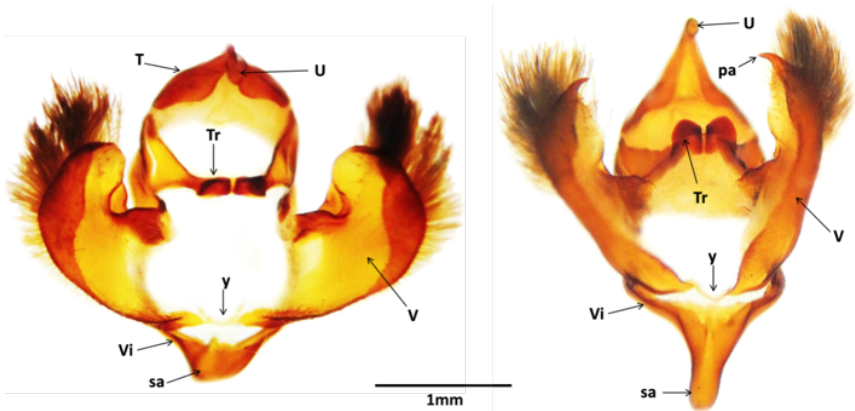
pa: proceso apical de la valva; sa: saccus; T: tegumen; Tr: transtilla; U: uncus; V: valva; Vi: vinculum; y: yuxta.
