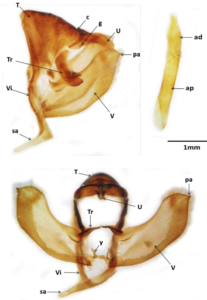
Fig. K. Fountainea nessus (Latreille)
