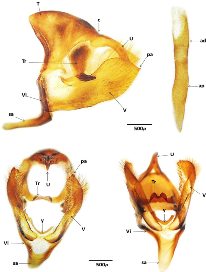
Fig A. Muysbondtia tyrianthina (Salvin & Godman)
