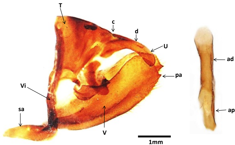
Fig. 10. Polygrapha cyanea silvaorum (Constantino & Salazar)
