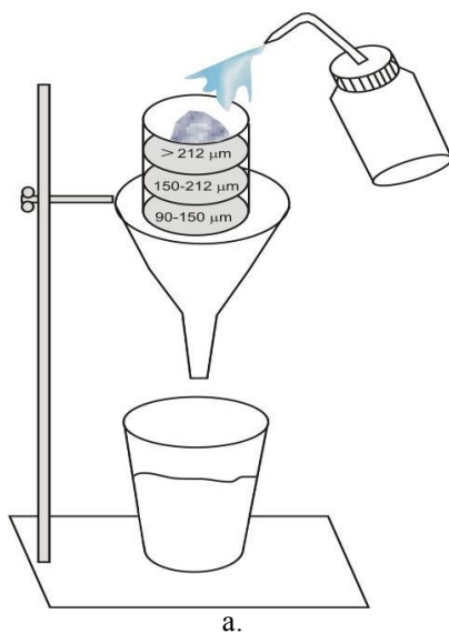
Figura 6. a. Esquema de montaje para tamizado en húmedo; b. Foto de montaje para tamizado en húmedo
