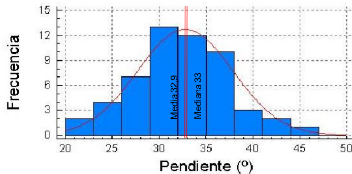
Figura 10. Rango de pendientes
