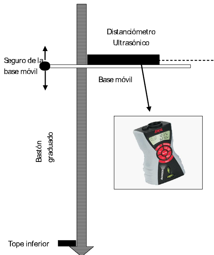
Figura 6. Esquema del distanciamiento
