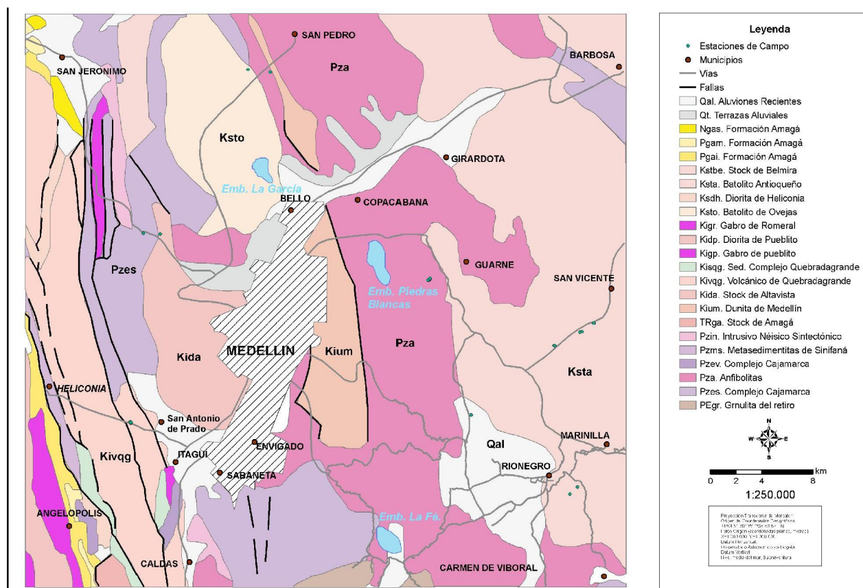
Figura 2. Mapa geológico.
