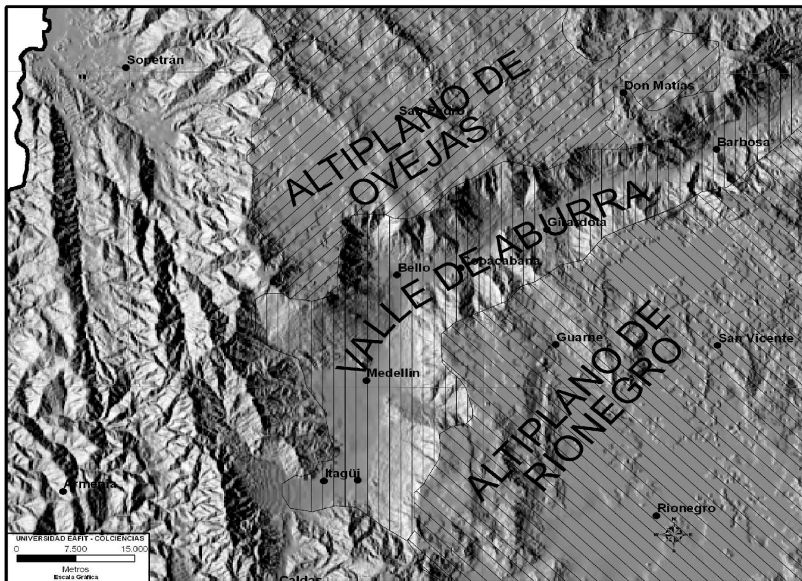
Figura 3. Geomorfología de la zona.
