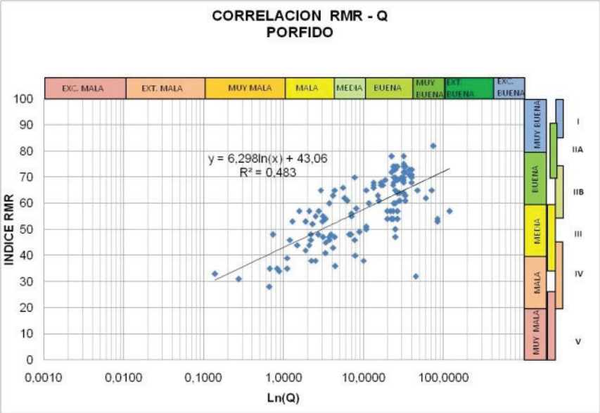
Figura 12. Correlacion LnQ-RMR en el cuerpo pórfido.
