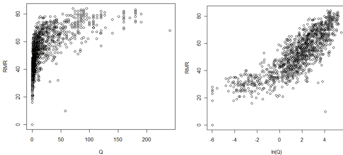
Figura 5. a) Relación entre Q y RMR. b) Relación entre el RMR y la transformación logarítmica de Q.
