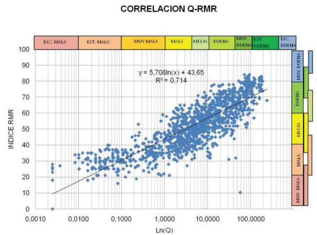
Figura 7. Correlación general en el TPL.
