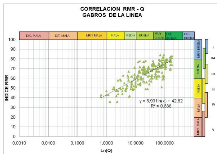
Figura 11. Correlacion LnQ-RMR en los Gabros de La Linea.
