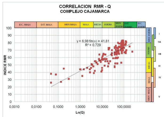
Figura 10. Correlacion LnQ-RMR en el Complejo Cajamarca.
