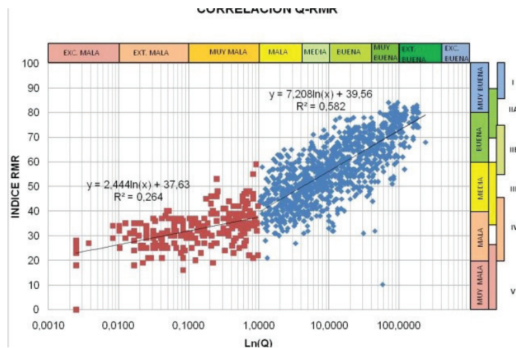
Figura 8. Correlación LnQ-RMR para Q menor y mayor a 1.
