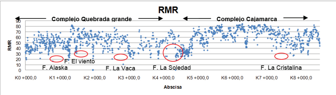
Figura 3. Valores de la clasificación RMR en el terreno atravesado por el Túnel Piloto de La Línea, son señaladas algunas fallas geológicas.
