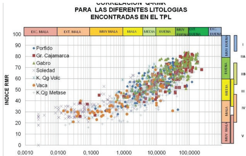
Figura 6. Relación entre el Q y el RMR en las principales unidades litológicas.
