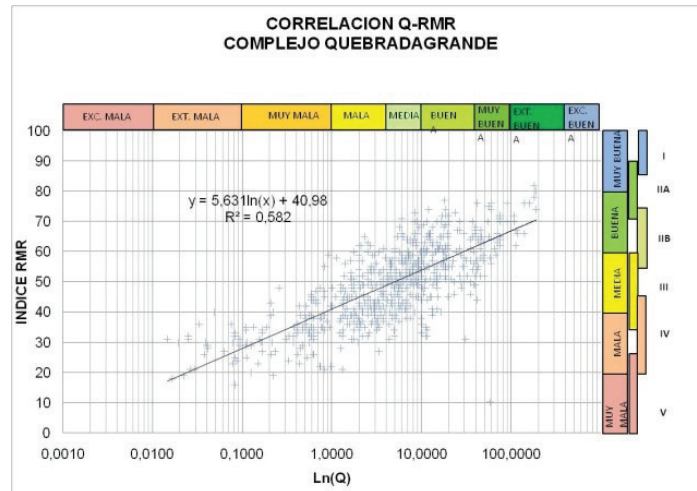
Figura 9. Correlacion LnQ-RMR en el Complejo Quebradagrande.
