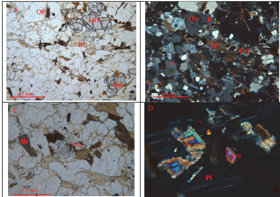
Figura 3. GZ-6782 (900798). Esquisto de Qtz-Pl-Kfs-Bt con granate. Escala gráfica, aumento 4x. A y C) Nicols paralelos. B y D) Nicols cruzados. Textura granolepidoblástica. Compuesta, por plagioclasa (Pl), cuarzo (Qtz), feldespato potásico y biotita (Bt), con granate (Grt). C) Nicols paralelos objetivo 10X circosnes tamaño 83 \mu m. D) Nicols cruzados, objetivo 25X.
