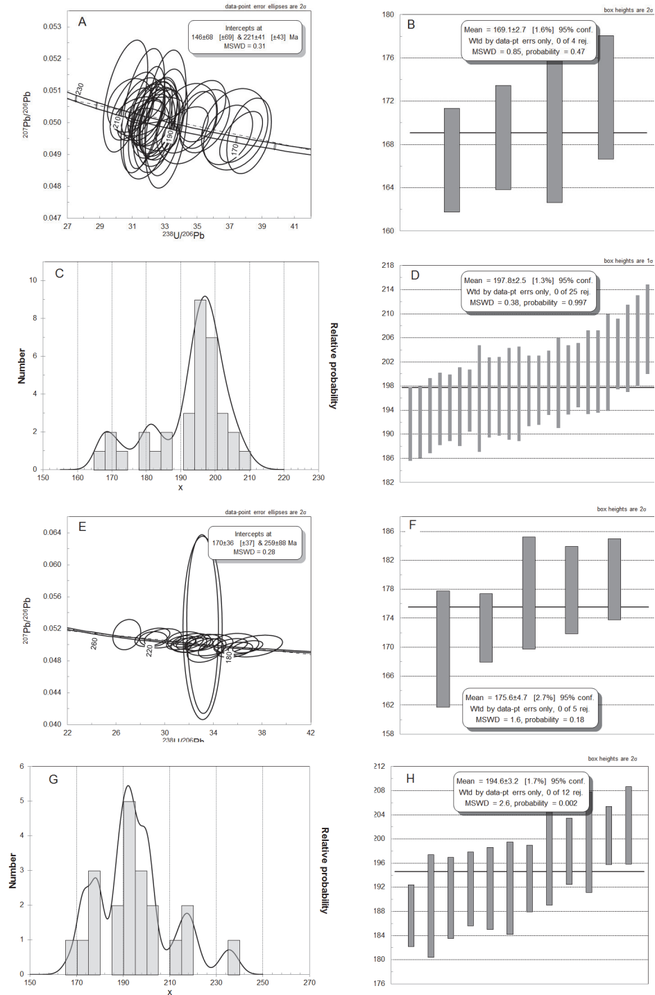
Figura 19. , B, C, D) Diagramas concordia, gráfico de probabilidades y cálculo de la de la edad media y desviación estándar para las edades U-Pb de la muestra GR-6596. E, F, G, H) para la de la muestra GR-6597.
