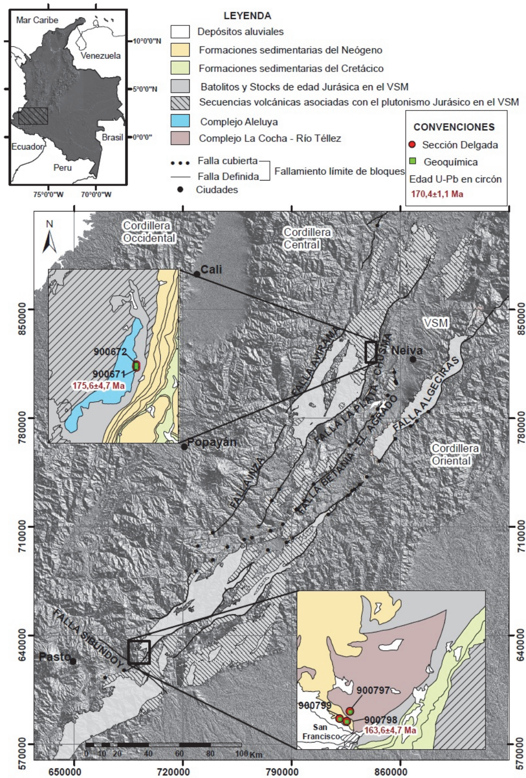
Figura 1. Localización de los complejos Aleluya y La Cocha – Río Téllez. Fuente: Los autores.
