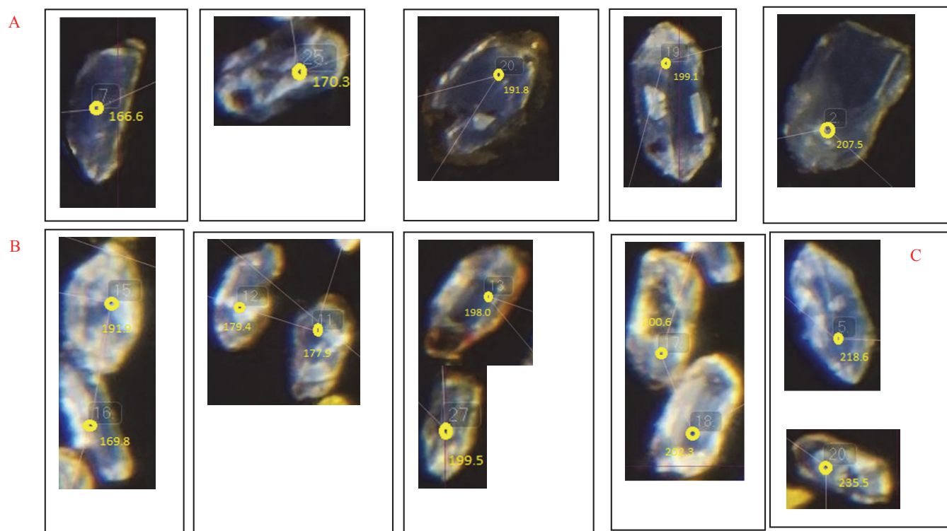
Figura 17. A) Imágenes de catodoluminiscencia de circones de las muestras GR-6596. B) GR-6597. C) circones heredados en GR-6597.
