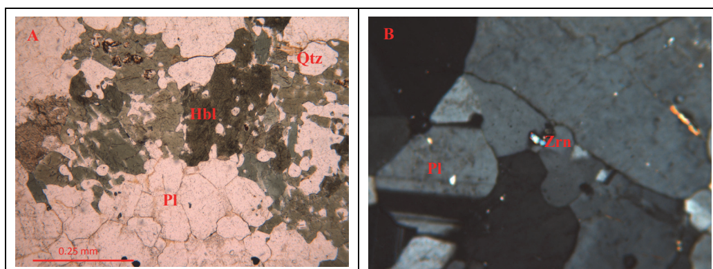
Figura 6. A) Aspecto microscópico de la muestra GR-6596 (IGM-900671). A) Nicols paralelos. Granofels de Pl-Qtz y Hbl. Escala gráfica, objetivo 4x. Cristales xenoblásticos de plagioclase (Pl), cuarzo (Qtz) y hornblenda (Hbl). B) Nicols cruzados, objetivo 10x cristal de circón (Zrn), tamaño 34 \mu\text{m} . Fuente: Los autores
