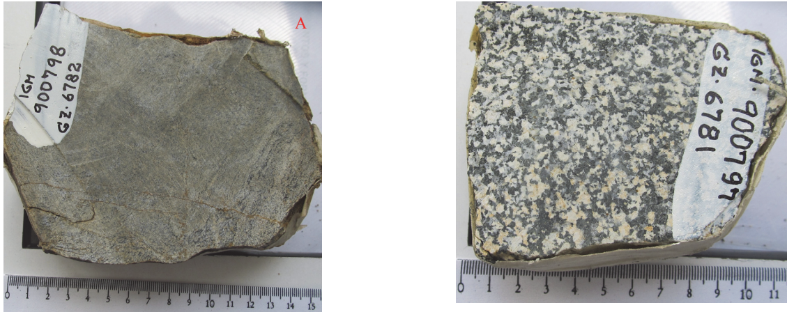
Figura 2. Aspecto macroscópico de las muestras 900798 (esquisto) y 900797 (granofels). Fuente: Los autores
