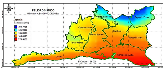
Figura 10. Imagen del modelo de peligrosidad sísmica provincia Santiago de Cuba.
