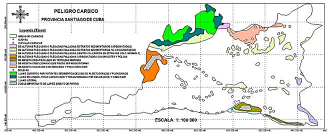
Figura 22. Imagen del mapa de desarrollo cársico o amenaza cársica.
