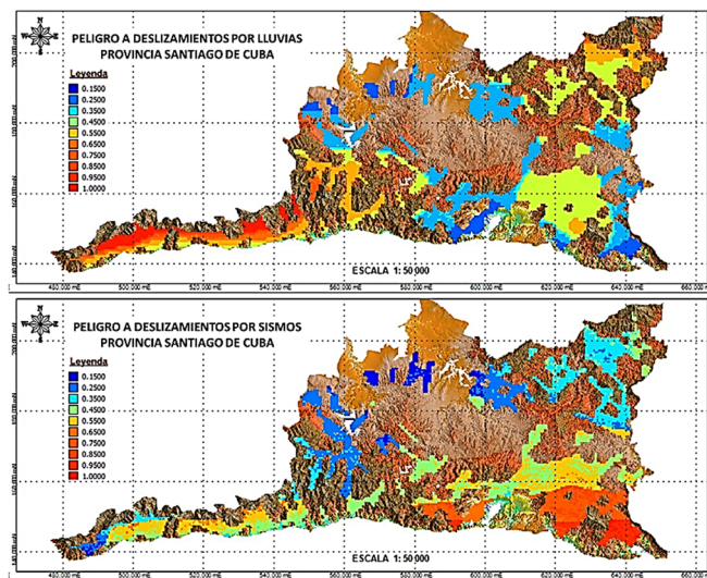
Figura 21. Imagen de los modelos de peligro a deslizamientos por lluvias (arriba) y sismos (abajo) de la provincia Santiago de Cuba.
