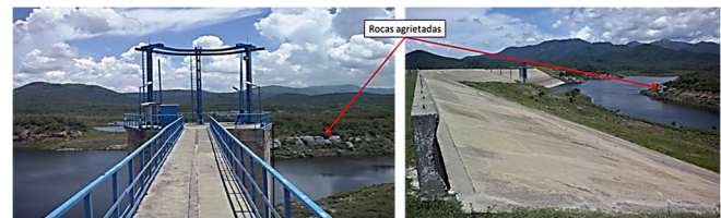
Figura 23. Imágenes de la presa Parada, señalándose el alto agrietamiento primario producto a la carsificación acelerada por los procesos microsísmicos regionales presentes en Santiago de Cuba.
