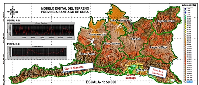
Figura 4. Imagen del Modelo Digital del Terreno (MDT) de la provincia Santiago de Cuba, significando su relieve.
