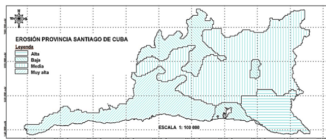
Figura 16. Imagen del modelo de erosión fluvial de la provincia Santiago de Cuba.
