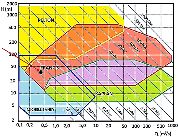
Figura 11. Abaco para determinar el tipo de turbina a emplear según cálculos iniciales, señalando la ubicación de selección primaria. Fuente: ESHA, 2006.
