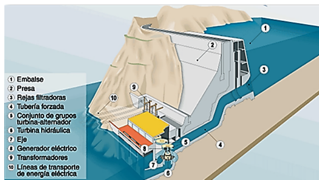
Figura 2. Esquema clásico de una central hidroeléctrica aguas debajo de una represa.
