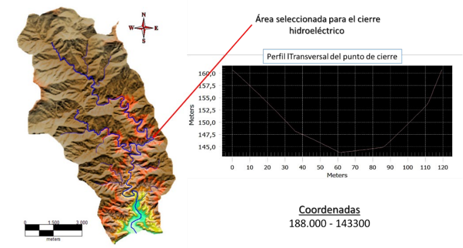
Figura 9. Área seleccionada para el cierre hidroeléctrico mostrando un perfil transversal.
