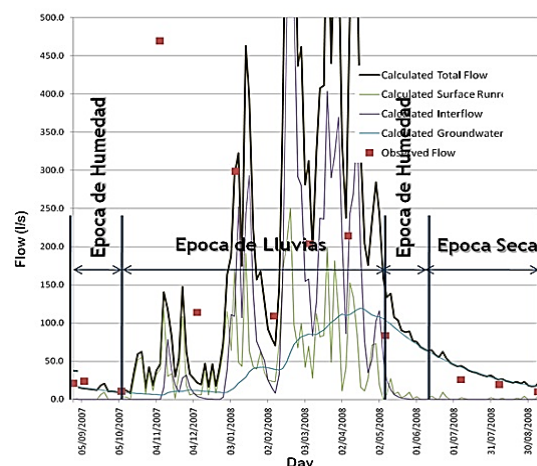
Figura 4. Ejemplo que se muestra en el método de “Modelamiento hidrológico distribuido” para determinación de caudales en la época húmeda y época seca con la curva de recesión luego del de las lluvias.
