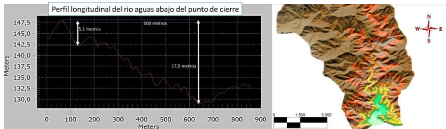
Figura 10. Perfil longitudinal del río aguas abajo del punto de cierre.
