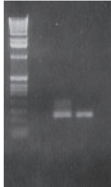
Figura 1. Amplificación por PCR del gen B1 específico de Toxoplasma gondii . Carril 1: marcador de peso molecular 1 kb ADN Ladder (Gibco BRL); carril 2: control negativo; carril 3: control positivo cepa RH; carril 4: cepa CIBMUQ/HDC. Se observa la amplificación de 2 fragmentos de 196 y 97 pb para el control positivo y un fragmento de 97 pb para la cepa CIBMUQ/HDC. Los productos se visualizaron en un gel de agarosa al 1% teñidos con bromuro de etidio.
