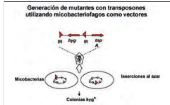
Figura 4. Inserción génica con transposones. Un transposón con un gen determinante de resistencia a la higromicina ( hyg ), las secuencias invertidas IR y el gen de la transposasa A ( tnpA ) se introducen en las micobacterias por medio de transducción utilizando un micobacteriófago. La integración del transposón ocurre al azar y genera mutantes en diferentes genes que se pueden seleccionar en medio con higromicina.
