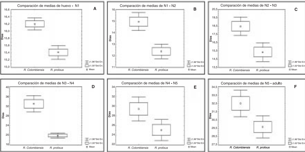
Figura 1. Comparación entre las medias del tiempo (días) de eclosión A (huevo-N1) y de muda de cada estadio de desarrollo (B: N1-N2, C: N2-N3, D: N3-N4, E: N4-N5 y F: N5-adulto) con sus respectivos intervalos de confianza de 95% para Rhodnius colombiensis y Rhodnius prolixus .
