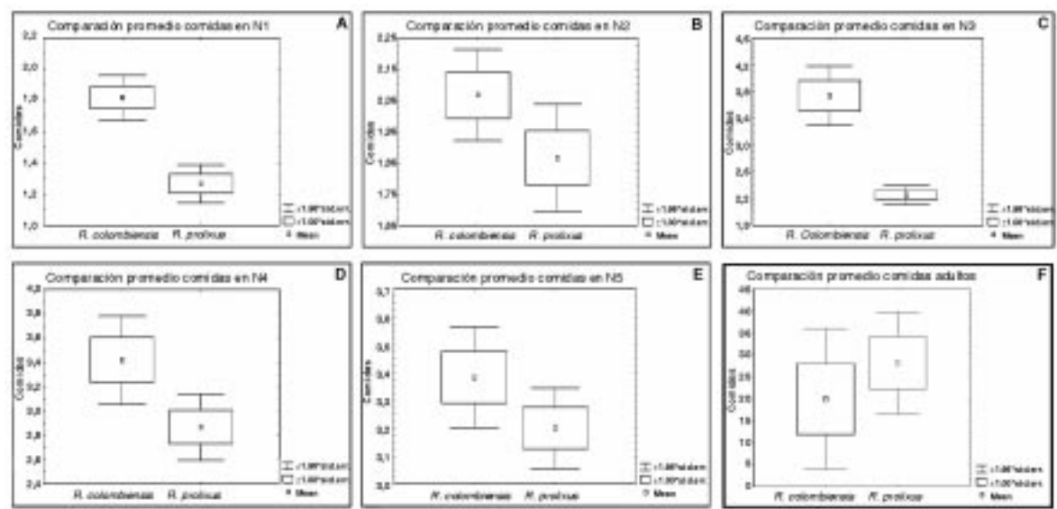
Figura 2. Comparación entre las medias del número de comidas y los intervalos de confianza de 95% para cada uno de los estadios de desarrollo (A: N1, B: N2, C: N3, D: N4, E: N5, F: adulto) para R. colombiensis y R. prolixus .
