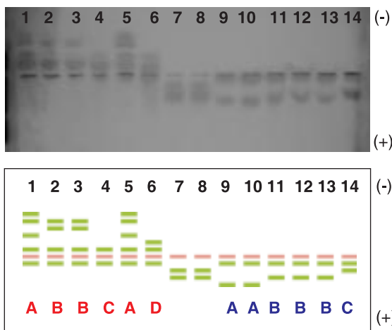
Figura 1. Electroforesis en gel delgado de almidón al 8% de hemoproteínas salivares de R. prolixus (canaletas 1 a 6), R. pallescens (canaletas 7 y 8) y R. colombiensis (canaletas 9 a 14). El panel inferior de la figura corresponde a un diagrama que representa las bandas del panel superior.
