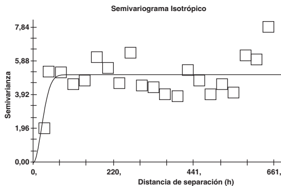
Figura 2. Semivariograma isotrópico calculado para el índice de recipientes
