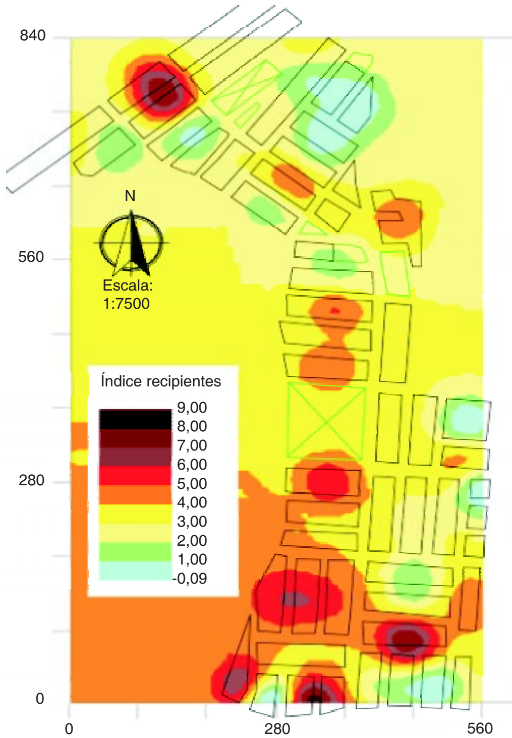
Figura 3. Representación gráfica bidimensional del kriging de la variable índice de recipientes.
