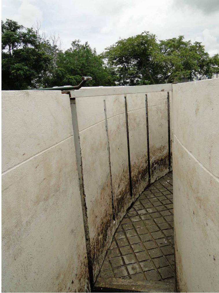
Figura 3. Las mangas de conducción deben tener paredes sólidas para evitar las distracciones de los animales.
