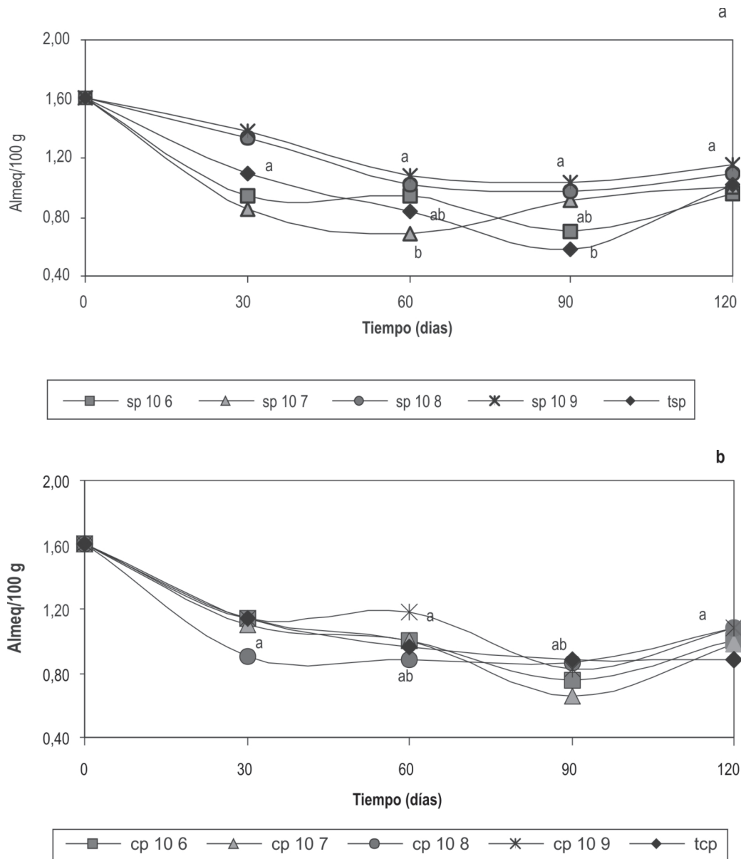
Figura 5. Variación en la concentración de aluminio de un Ultisol, con aplicación de B. subtilis en concentraciones de 10^6 , 10^7 , 10^8 , 10^9 ufc, a) sin planta (sp) y b) con planta (cp). Letras iguales en las gráficas significan que no hubo diferencias significativas con un \alpha de 0,05 en la prueba de comparación de medias de Duncan.
