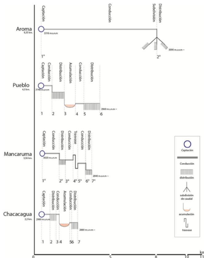
Imagen 6. Diagrama lineal de la distribución del agua en los espacios hidráulicos que forman los cuatro canales matrices
