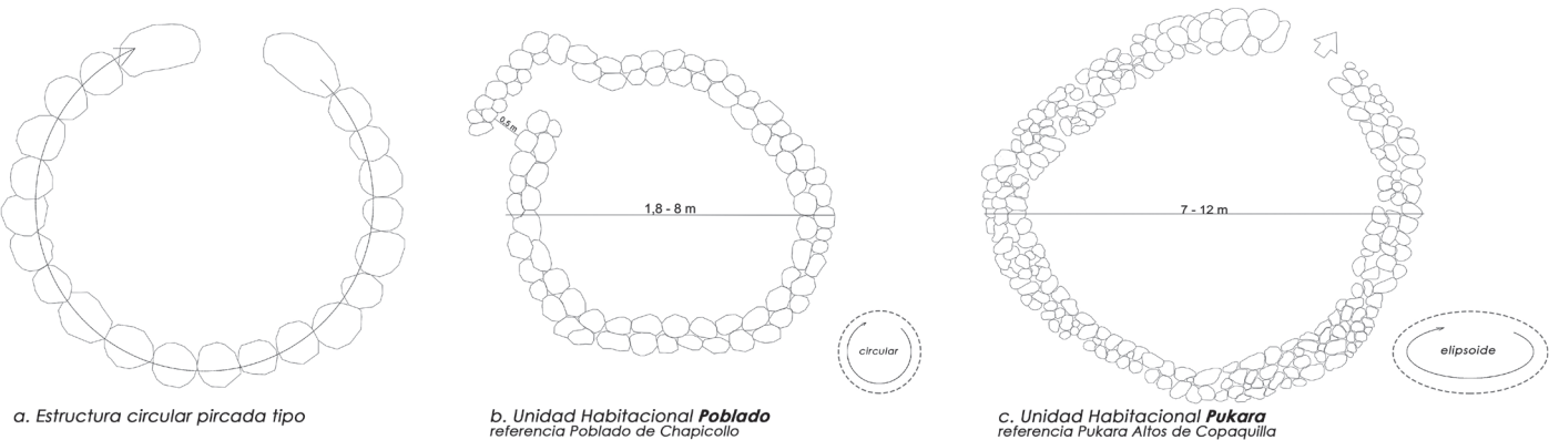
Figura 4. Tipos y formas constructivas
