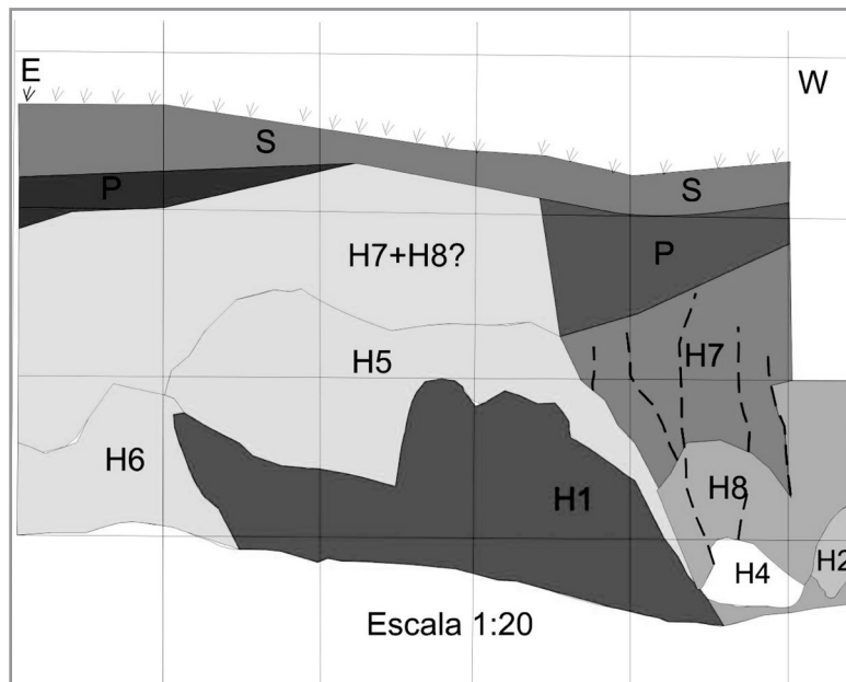
FIGURA 2. Levantamiento paleosísmico trinchera Portal W
