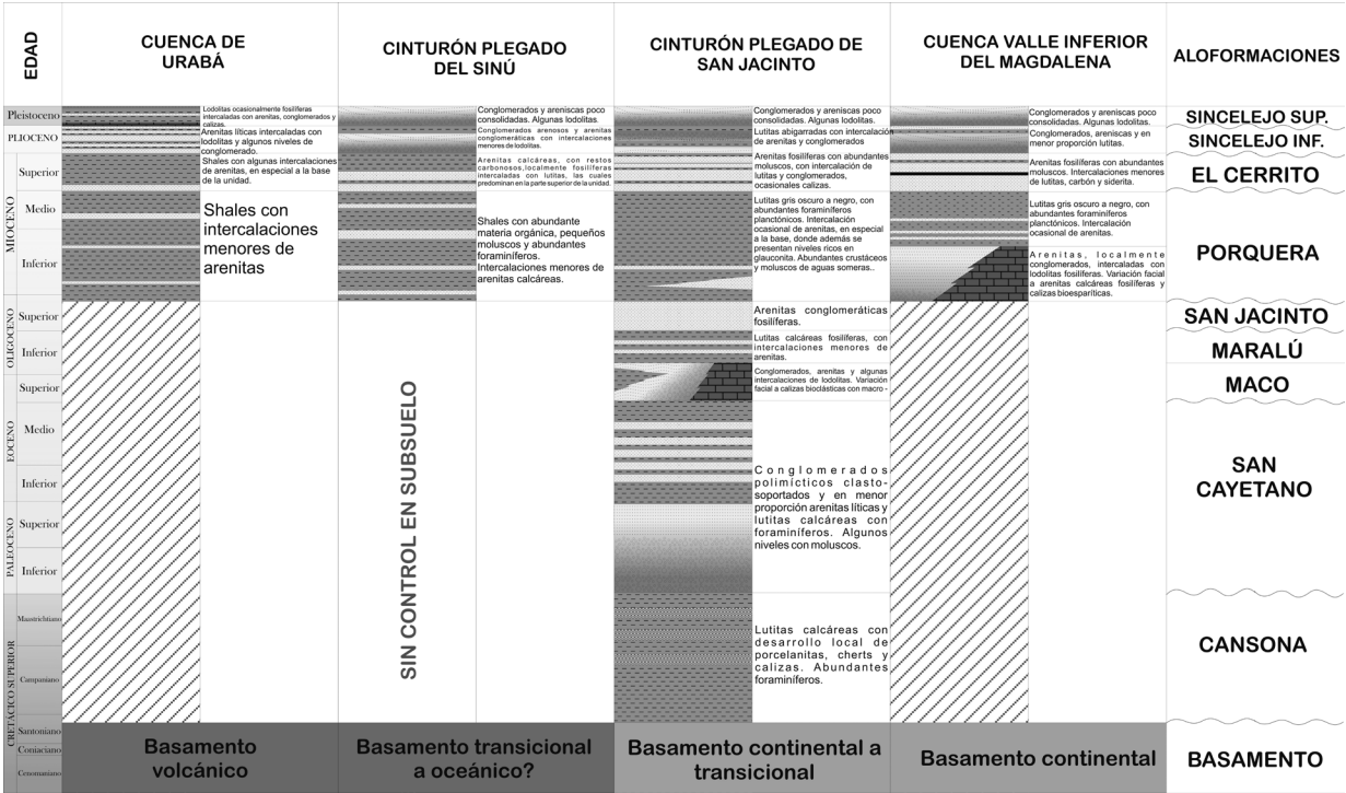
FIGURA 2. Columna generalizada del área de estudio.
