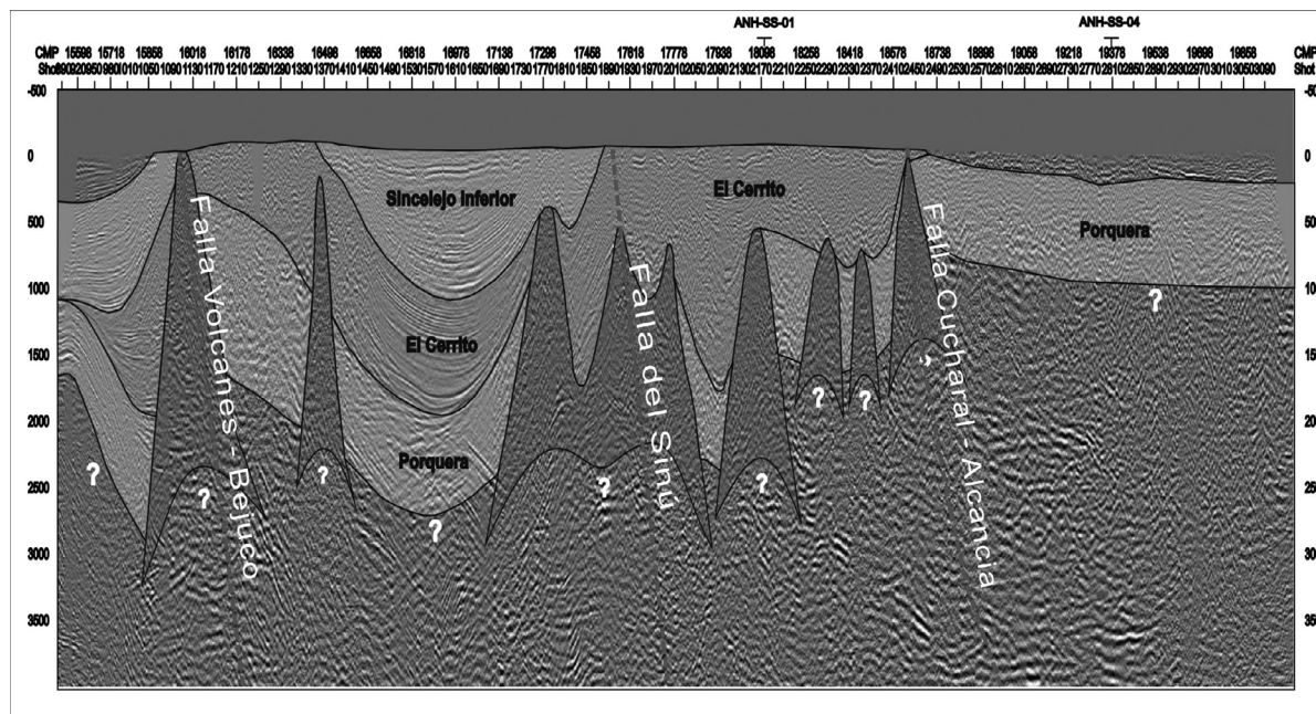
FIGURA 7. Línea ANH 2005-02, mostrando los tipos de plays observados en la sísmica y que no han sido probados hasta el momento con los pozos perforados en el área del Cinturón Plegado del Sinú.
