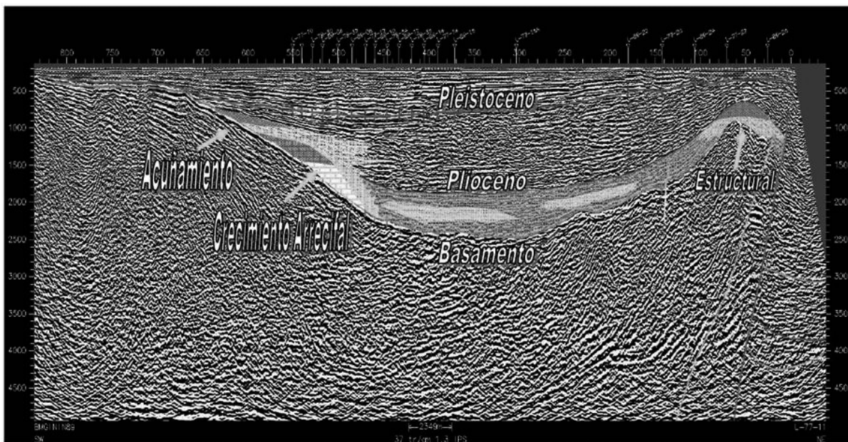
FIGURA 8. Línea sísmica del área de la Cuenca de Uribá, mostrando los tipos de plays antes mencionados. A la derecha un pliegue asociado a fallas inversas, y a la izquierda el acuñamiento o pinchamiento de sedimentos contra el basamento y el desarrollo de crecimientos arrecifales. Halliburton, 2007.
