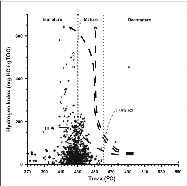
FIGURA 3. Diagrama de Van Krevelen (modificado) de la Cuenca Valle Inferior del Magdalena que muestra la madurez y el tipo de kerógeno (kerógeno tipo III: materia orgánica hímica-terrestre). Universidad de Caldas, 2008.
