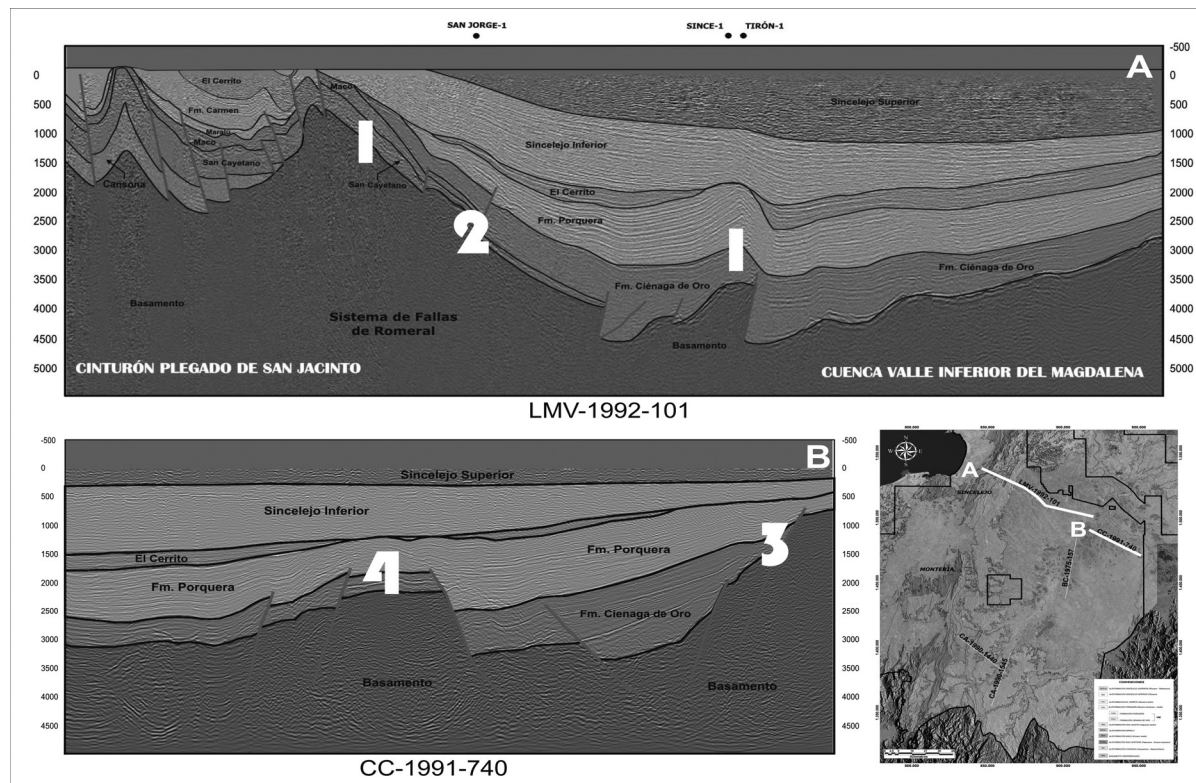
FIGURA 4. Tipos de plays en la Cuenca Valle Inferior del Magdalena. Universidad de Caldas, 2008.
