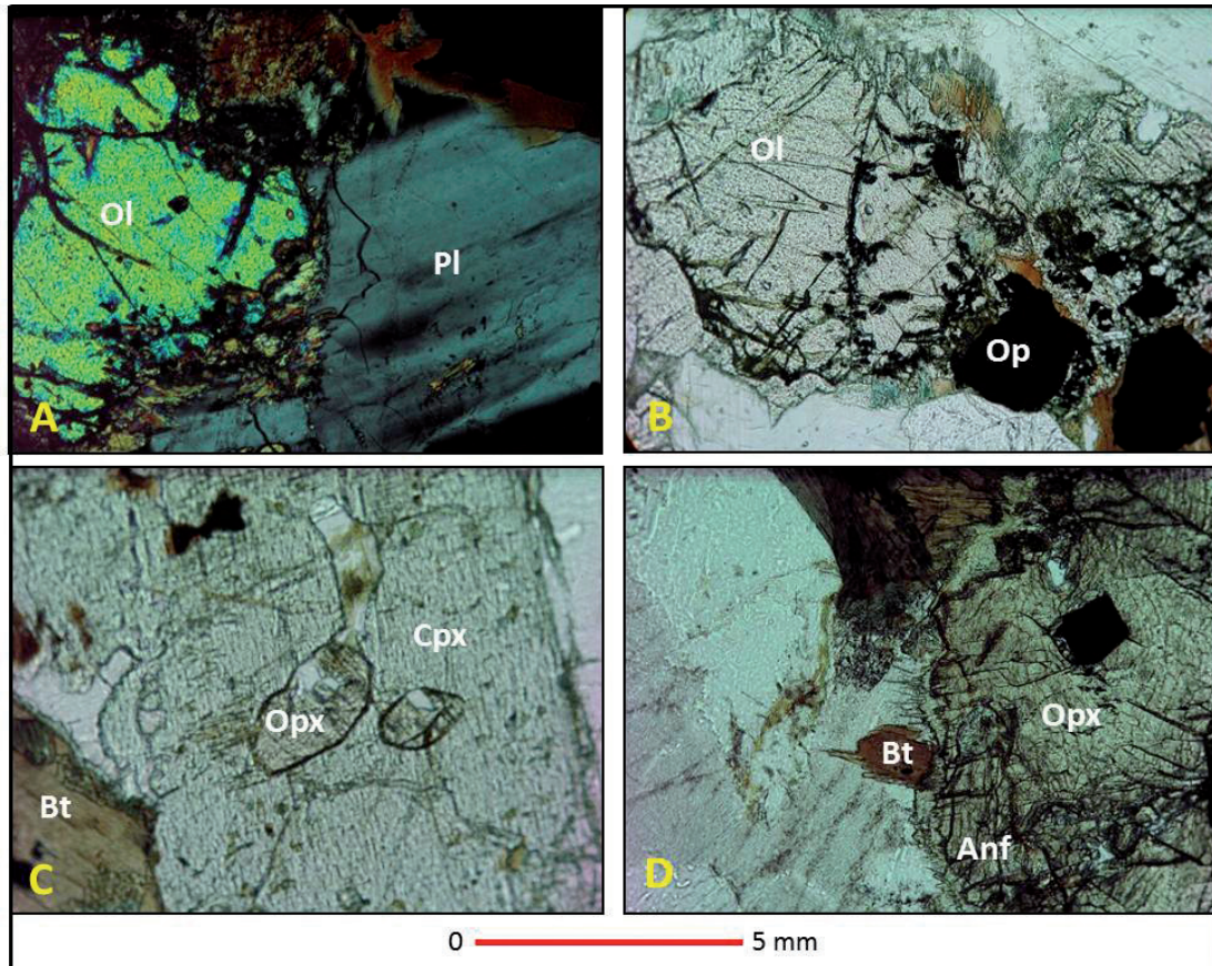
FIGURA 4. A) y B) Muestra 119058 10x cristales de olivino con fractura concoidea y acumulación de magnetita a lo largo de las fracturas, con corona de clinopiroxeno (Cpx) alterado a anfíbol uralítico. C) y D) Muestra 706806 10x, cristales de ortopiroxeno (Opx) incluidos en clinopiroxeno (augita) (Cpx).
