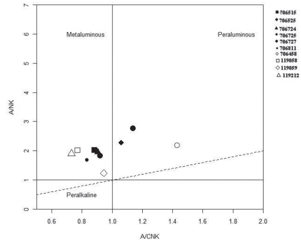
FIGURA 7. Diagrama de alcalinidad aluminosidad para la Granodiorita de Farallones.
