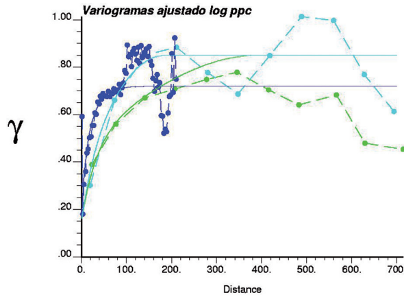
FIGURA 5. Variografía de la pérdida por calcinación.
