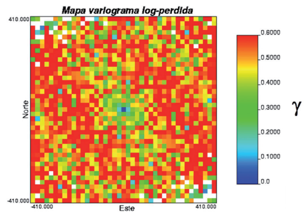
FIGURA 10. Dirección de anisotropía de la pérdida por calcinación.
