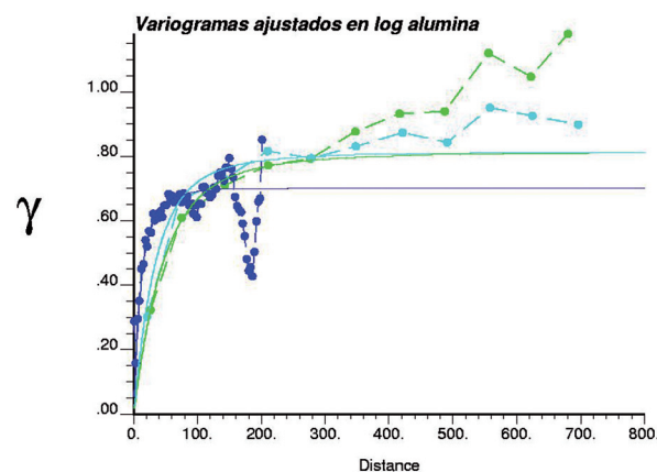
FIGURA 4. Variografía de la alúmina.
