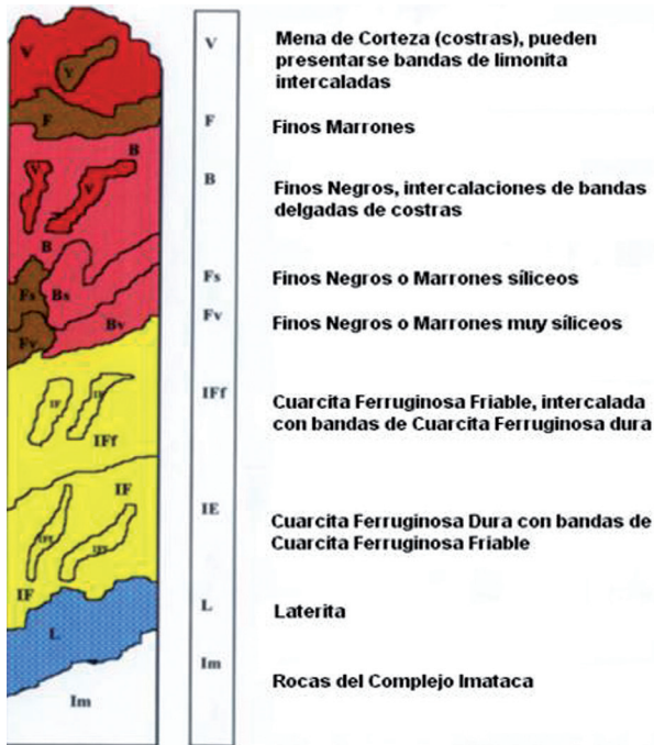
FIGURA 2. Corte litológico de los yacimientos de mineral de hierro. Tomado de C.V.G. Ferrominera Orinoco, C.A. (1991).
