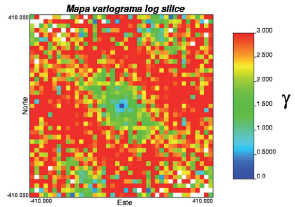
FIGURA 8. Dirección de anisotropía de la sílice.
