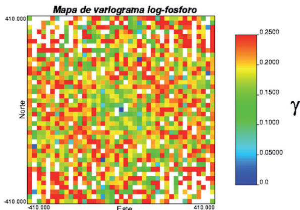
FIGURA 11. Dirección de anisotropía del fósforo.
