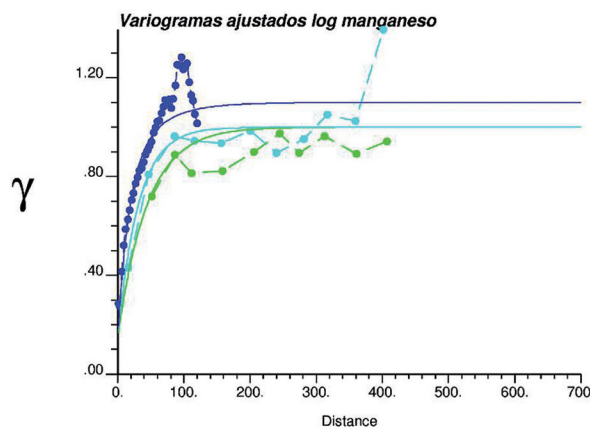
FIGURA 7. Variografía del manganeso.
