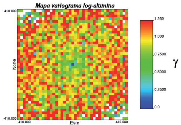
FIGURA 9. Dirección de anisotropía de la alúmina.
