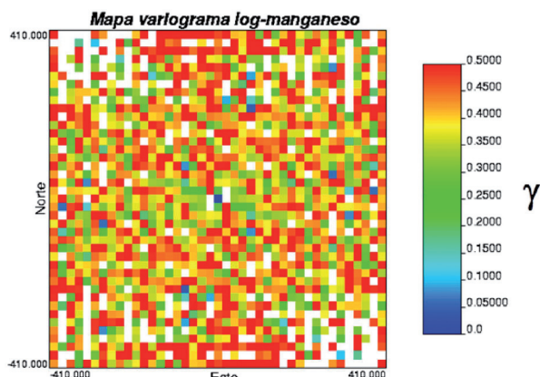
FIGURA 12. Dirección de anisotropía del manganeso.
