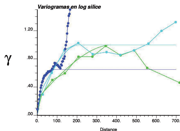
FIGURA 3. Variografía de la sílice.
