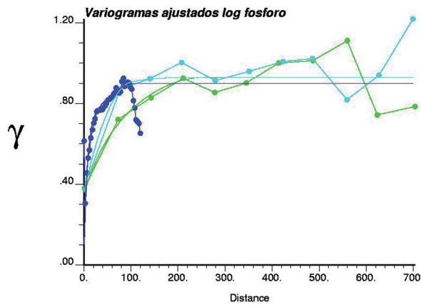
FIGURA 6. Variografía del fósforo.
