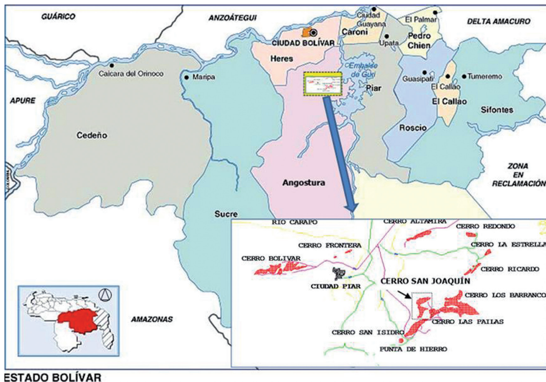
FIGURA 1. Mapa de ubicación del cerro San Joaquín. Modificado y ensamblado de Gobierno Bolivariano(S/F) y C.V.G. Ferrominera Orinoco, C.A. (1991).
