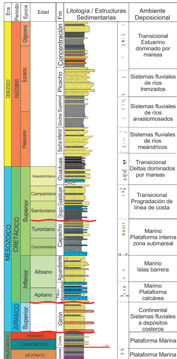
FIGURA 3. Columna estratigráfica generalizada de las unidades presentes desde el Devónico hasta el Oligoceno. Las líneas rojas irregulares corresponden a discontinuidades regionales y límites de secuencia. Modificado de Alarcón y Villar (2016).
