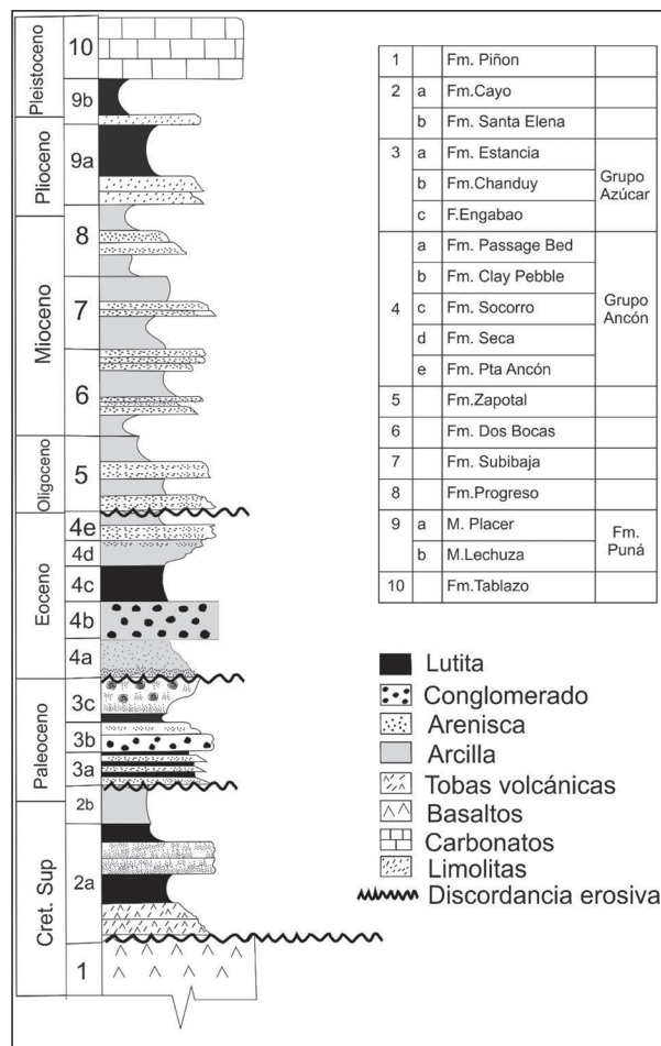
FIGURA 2. Columna Estratigráfica Progreso/Santa Elena integradas.
