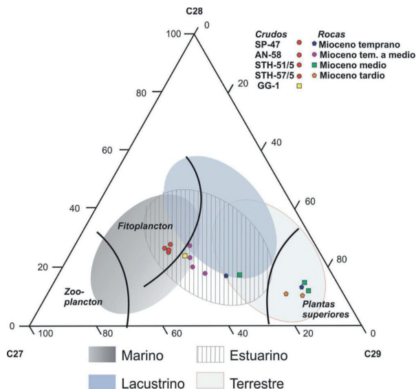
FIGURA 11. Diagrama triangular mostrando la contribución de los esteranos regulares \alpha\alpha\alpha y \alpha\beta\beta C_{27} , C_{28} y C_{29} . La interpretación paleoambiental y de fuente acorde a Huang y Meinschein (1979).
