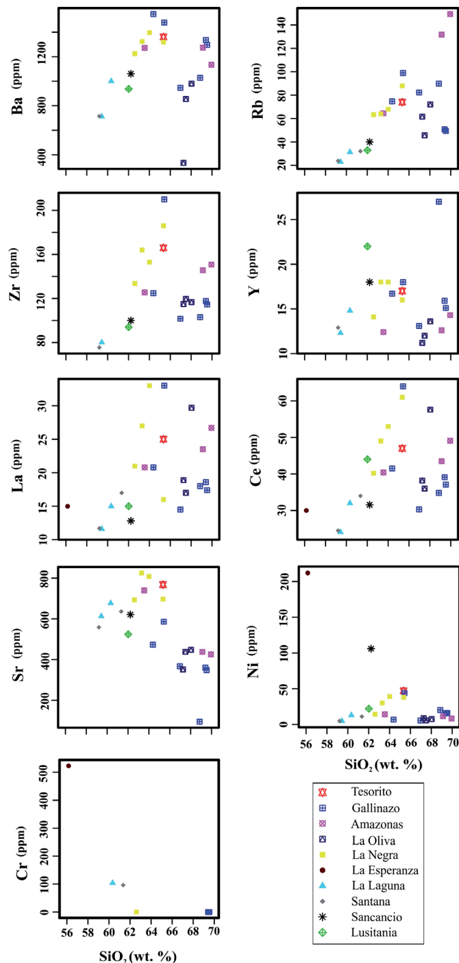
FIGURA 8. Diagramas de variación de elementos traza vs contenido de sílice para los volcanes del Campo Volcánico Monogenético Villamaria-Termes (CVMVT).
