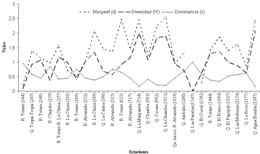
Figura 4. Variación espacial de los valores de riqueza de Margalef (D), diversidad de Shannon-Wiener ( H' ) y de dominancia de Simpson ( \lambda ) en la cuenca del río Totare durante febrero y mayo de 2007. Se indica la altitud de cada estación (m).
