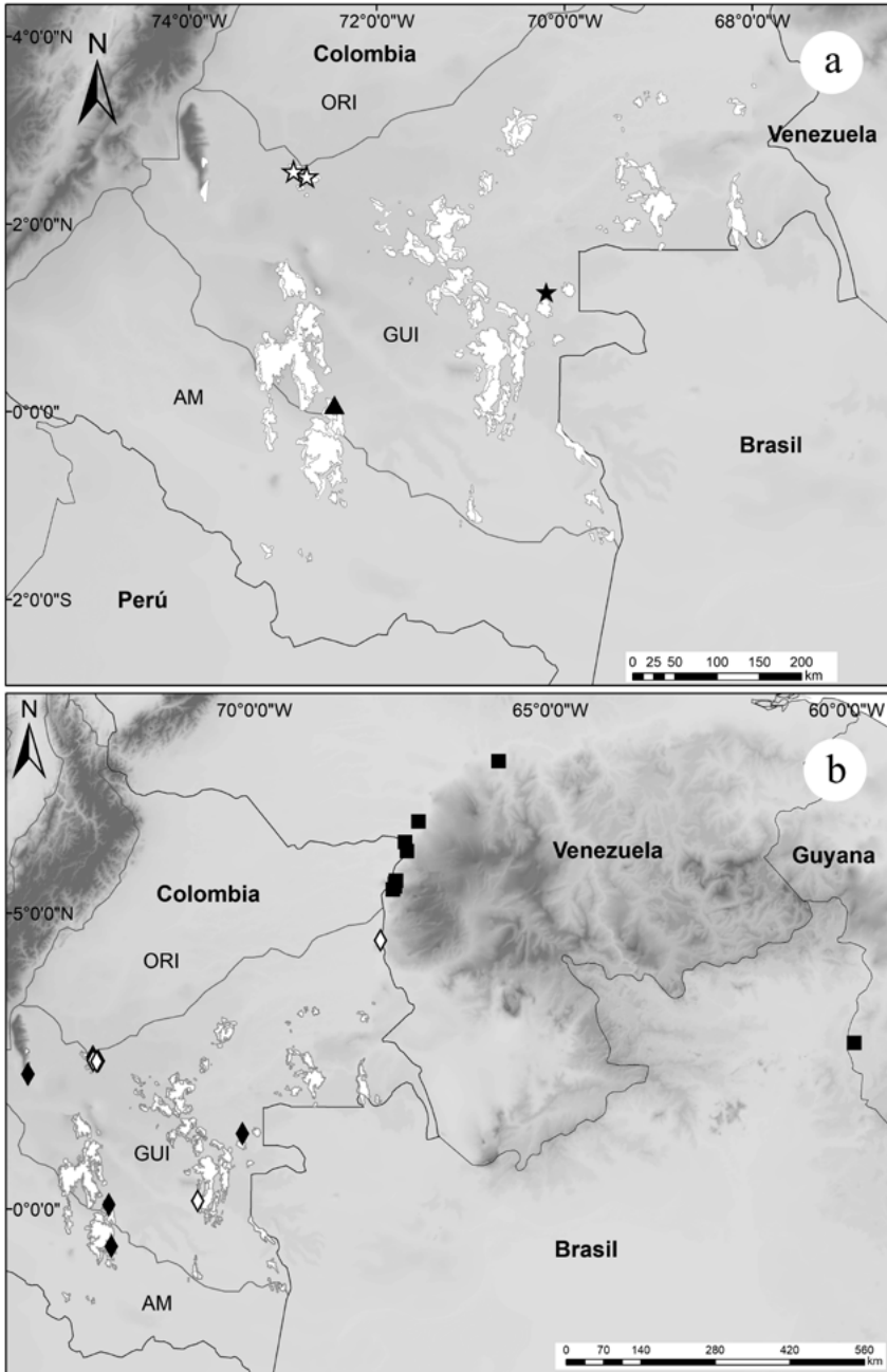
Figura 2. Distribución de a. Lonchorhina mankomara y Lonchorhina marinkellei ; y b. Lonchorhina orinocensis ; ORI = Llanos del Orinoco; GUI = Guayana; AM = Amazonía. Manchas en blanco representan la distribución de los inselbergs en la Orinoquía. Estrellas = localidades de L. marinkellei . Triángulo = localidad tipo de L. mankomara . Cuadrados= Localidades de L. orinocensis fuera de Colombia, Rombos = Localidades de L. orinocensis de Colombia. Símbolos negros: localidades extraídas de literatura. Símbolos blancos nuevas localidades de L. marinkellei y L. orinocensis .
