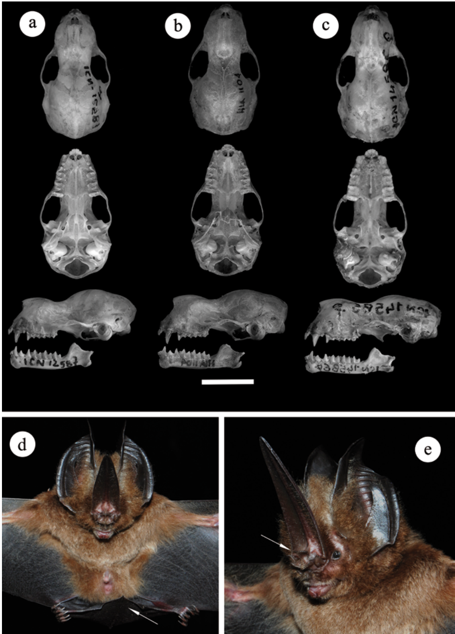
Figura 3. Estructuras comparadas de L. marinkellei y L. mankomara . a, b y c, comparación de las vistas dorsales, ventrales y laterales del cráneo, y vistas laterales de las mandíbulas de: a. L. marinkellei de Mitú, Vaupés (Localidad tipo; ICN 12587); b. L. marinkellei de La Lindosa, Guaviare (ICN 22472, nuevo registro); y c. L. mankomara de Puerto Abeja, Caquetá (localidad tipo; ICN 14585). Escala = 10 mm; d y e. Caracteres externos de Lonchorhina marinkellei (ICN 23138): d. Imagen mostrando la extensión de la cola hasta el borde final del uropatagio. e. Detalle de la hoja nasal un poco mayor que la longitud de las orejas y la presencia de una sella larga con un tubérculo en forma de yunque.
