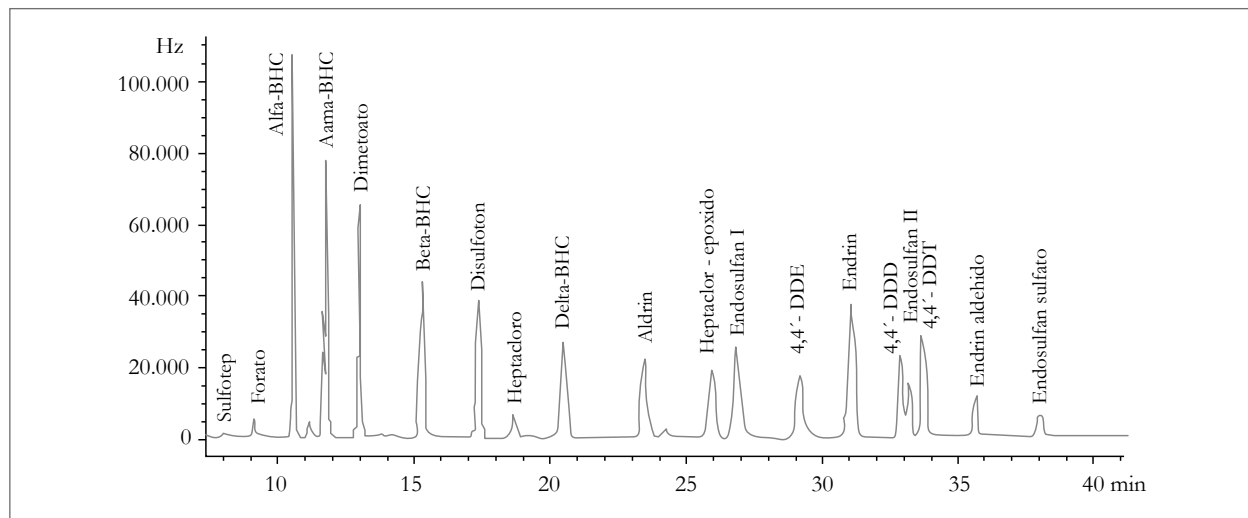
Figura 1. Cromatograma de la mezcla de estándares de plaguicidas OC y OF usados para la construcción de las curvas de calibrado por el método estándar externo.
