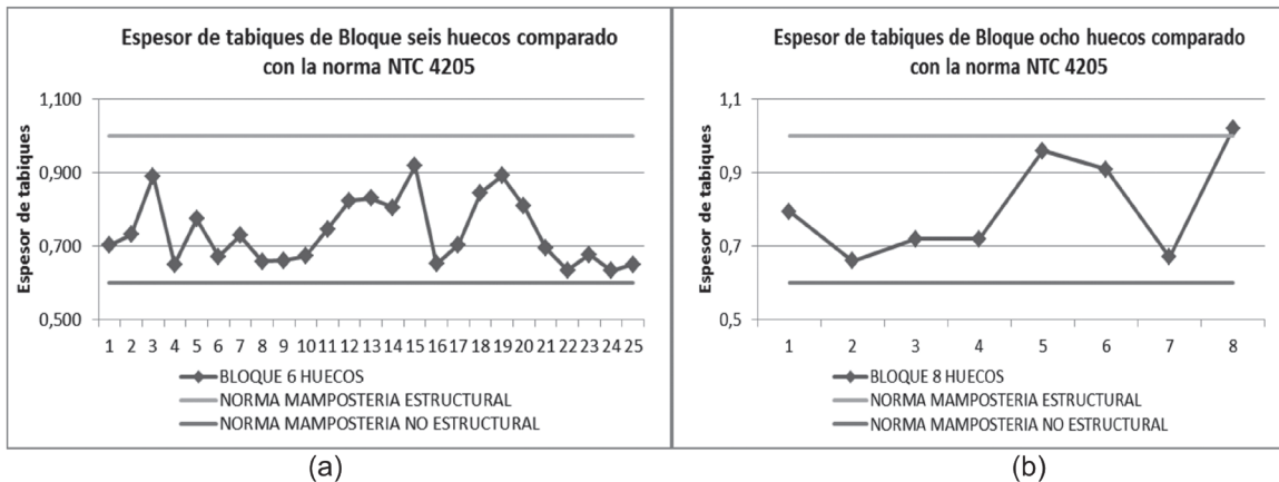
Figura 8. (a) Espesor de tabiques de bloques H10 seis huecos cuadrado. (b) Espesor de tabiques de los bloques H10 ocho huecos mixto.
