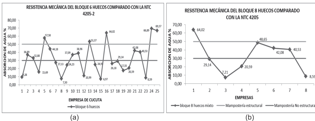
Figura 10. (a) Resistencia mecánica a la compresión de bloques H10 seis huecos cuadrado. (b) Resistencia mecánica a la compresión de bloques H10 ocho huecos mixto.
