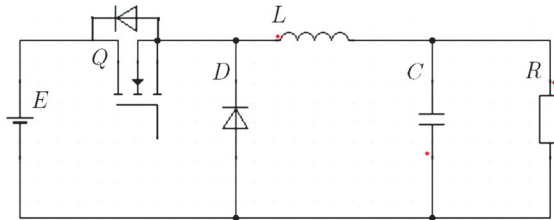
Figura 2. Convertidor Buck.
