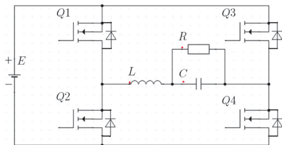
Figura 1. Puente completo en configuración H.
