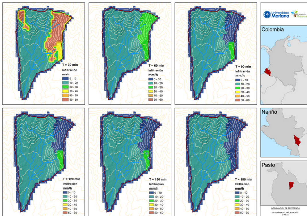
Figura 7. Resultados de simulaciones de infiltración de la microcuenca El Blanco
