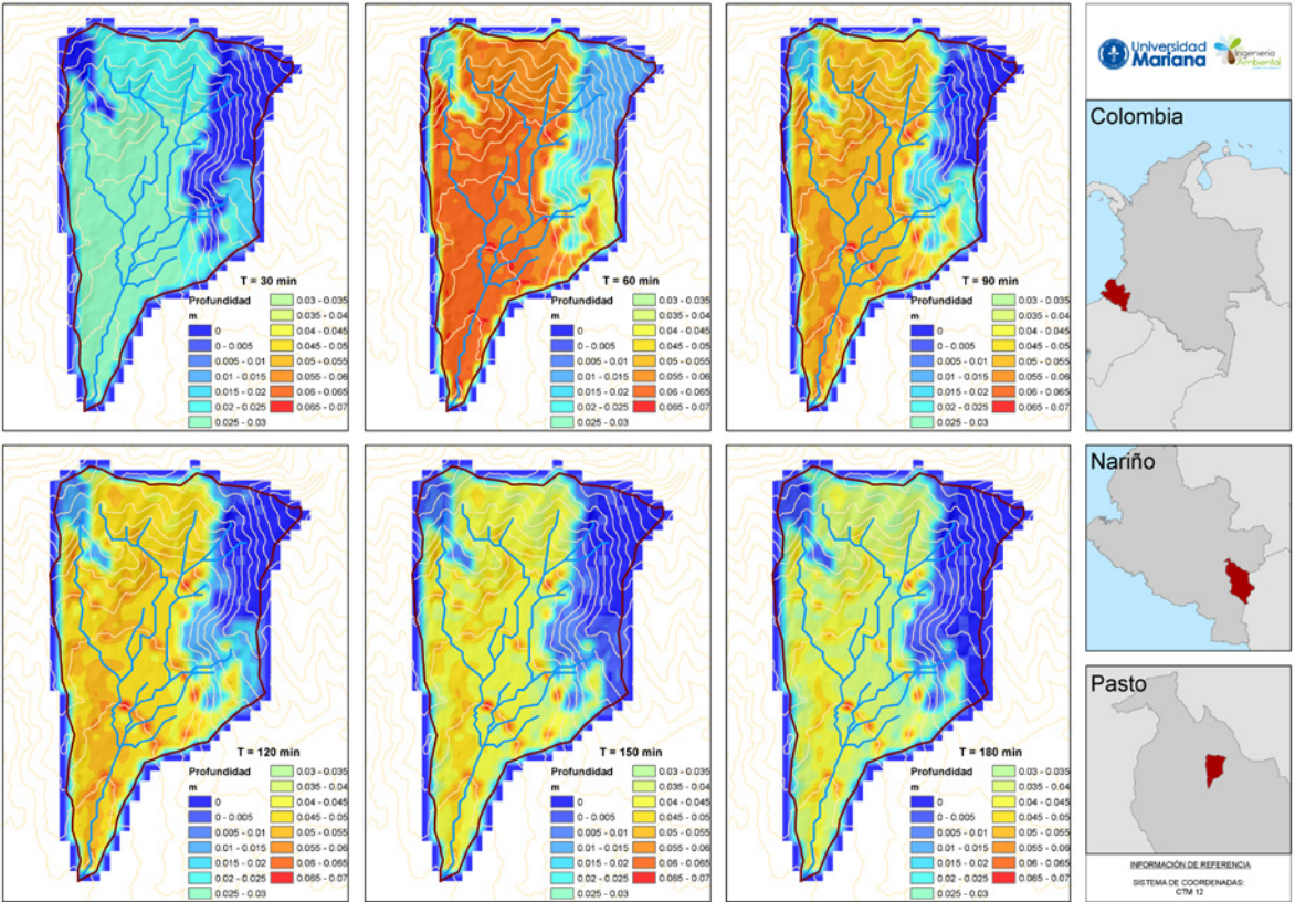
Figura 5. Resultados de simulaciones de profundidad de la microcuenca El Blanco
