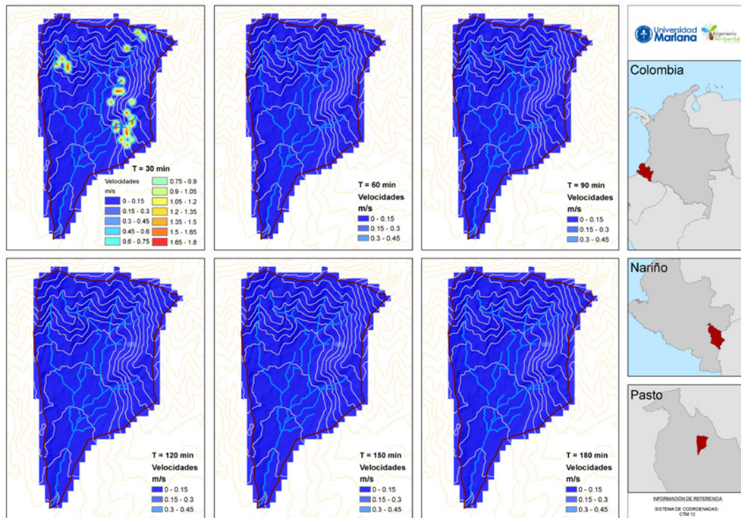
Figura 6. Resultados de simulaciones de velocidad de la microcuenca El Blanco
