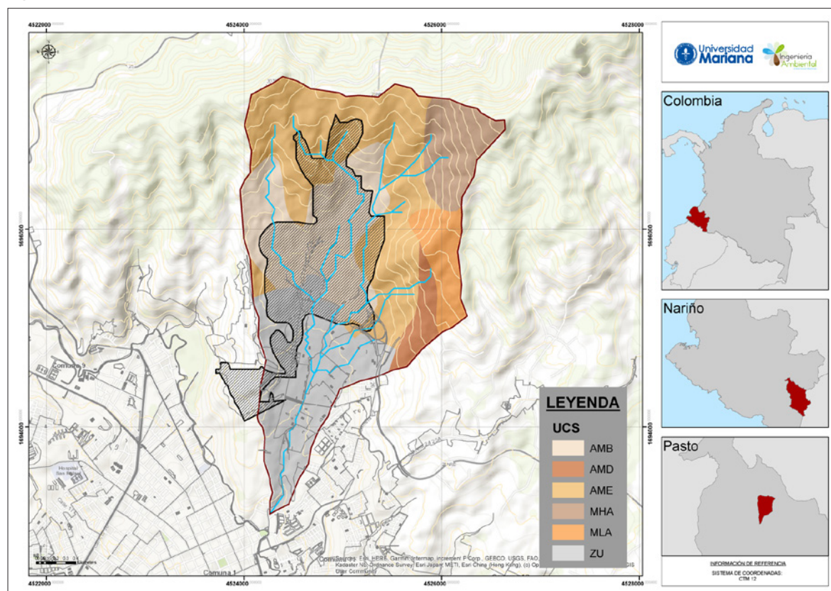
Figura 3. Consociaciones de suelos de la microcuenca El Blanco
