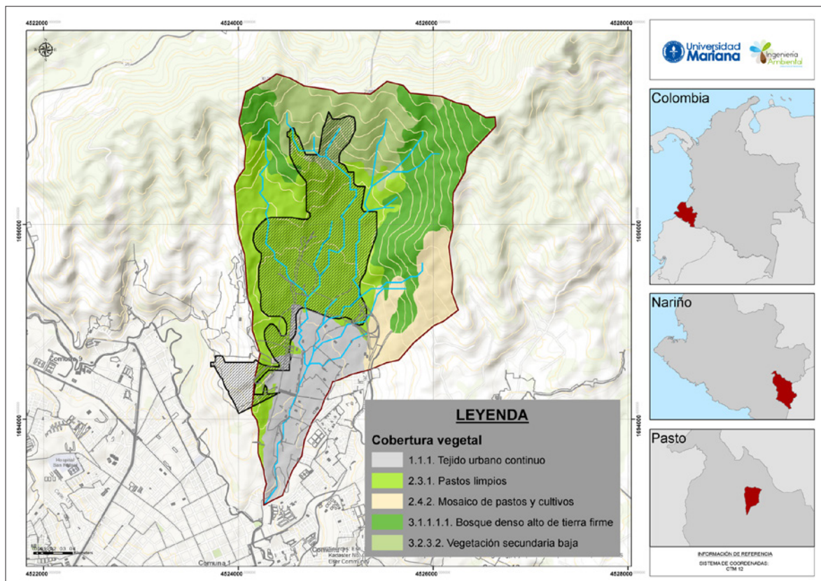
Figura 4. Mapa de coberturas de la microcuenca El Blanco
