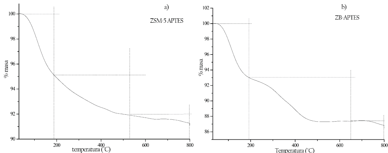
Figura 7. Análisis termogravimétrico de los materiales funcionalizados con APTES en: a) ZSM-5 y b) Z \beta -APTES.
