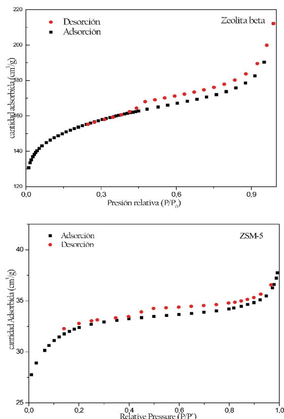
Figura 5. Isotermas de adsorción de N_2 para: a) Z \beta y b) ZSM-5.
