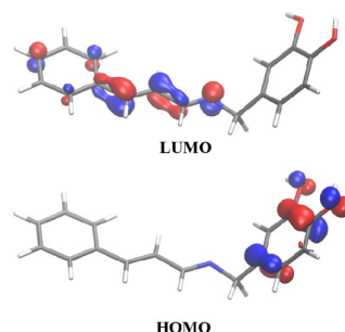
Figura 3. HOMO y LUMO, resultado del análisis de los orbitales de Kohn y Sham para la imina BS1-DA-CA.
