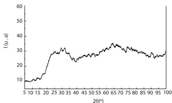
Figura 7. Espectro de DRX para el vidrio.
