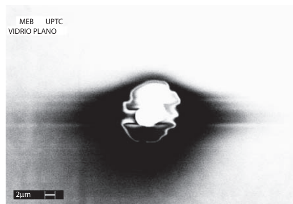
Figura 2. Infundido de sílice.
