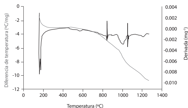
Figura 9. Diagrama DTA en muestra de vidrio.
