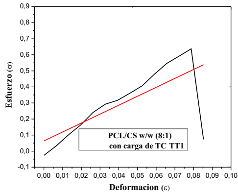
Figura 6. Curvas de tensión-deformación de las membranas electrohiladas de: PCL/CS w/w (10:1) con carga de TC (a) TT1, (b) TT2, (c) TT3 (d) TT4 y (e) PCL/CS w/w (8:1) con carga de TC TT1.
