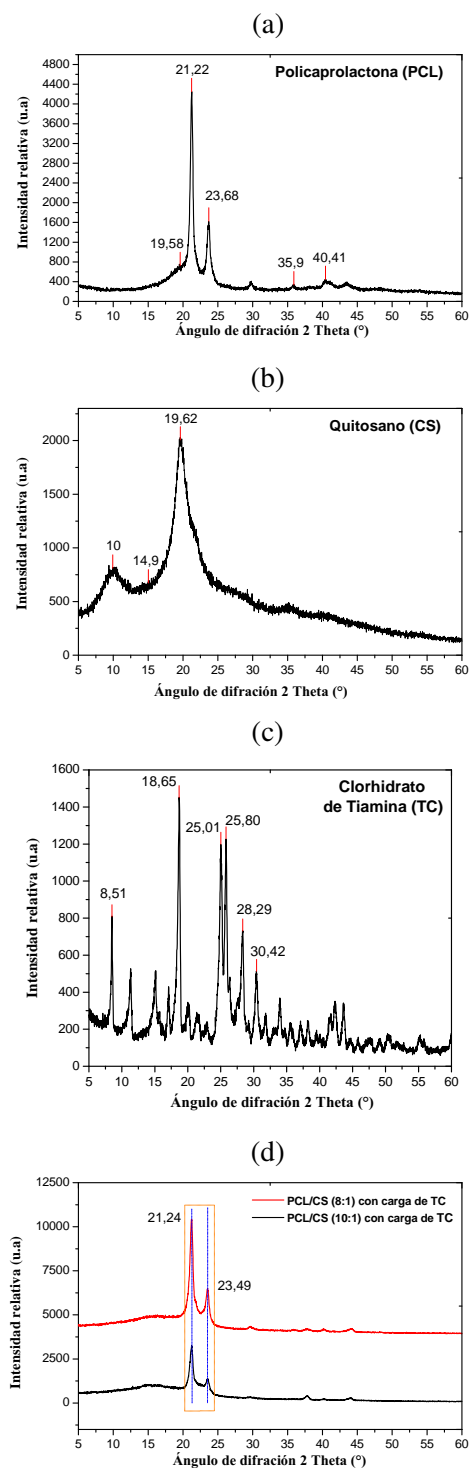
Figura 4. Difracción de rayos-X de: (a) Policaprolactona, (b) Quitosano, (c) Clorhidrato de Tiamina, (d) Membranas electrohiladas para estudios de la cinética de liberación.
