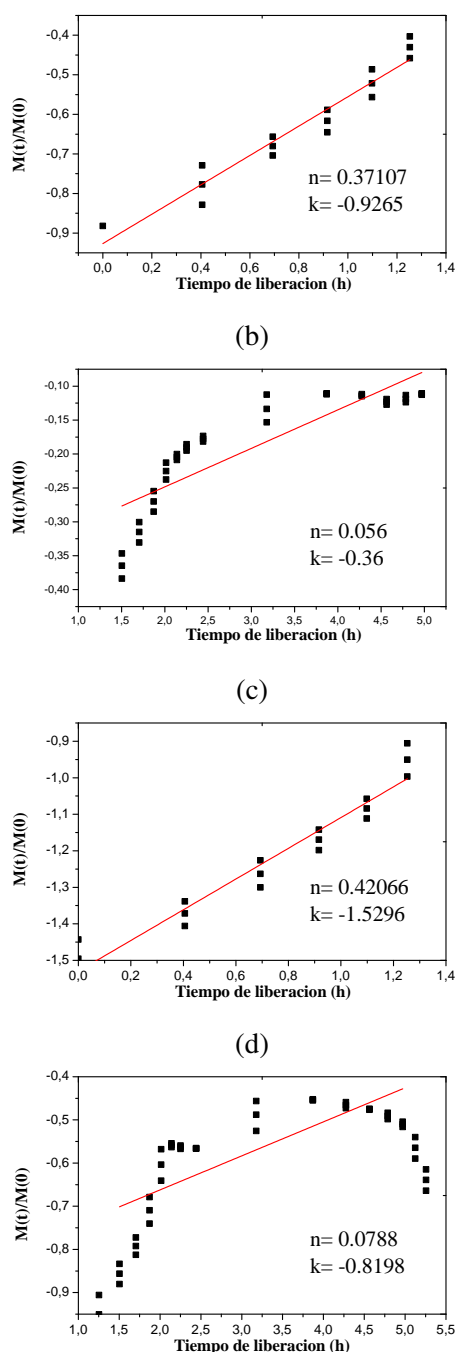
Figura 9. Perfil de liberación del clorhidrato de tiamina (a, b) PCL/CS w/w (8:1), (c, d) PCL/CS w/w (10:1).
