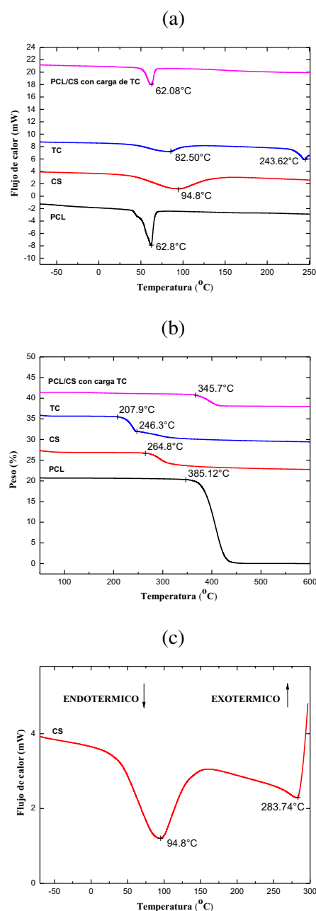
Figura 3. Termogramas de los materiales y la membrana PCL/CS w/w (8:1) con carga de TC en TFA/DCM v/v (4:1): (a) DSC, (b) TGA y (c) DSC del CS.
