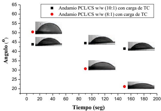
Figura 5. Medición de Ángulo de contacto vs Tiempo para las membranas electrohiladas de PCL/CS w/w (8:1) y (10:1).
