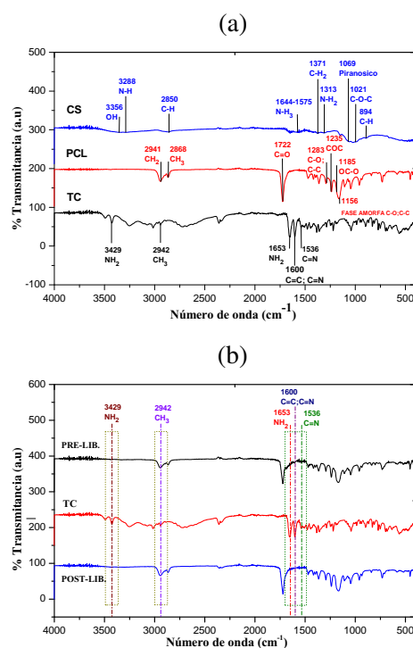
Figura 2. Espectros FTIR de: (a) reactivos puros y (b) membranas electrohiladas de PCL/CS pre y post-liberación de TC.
