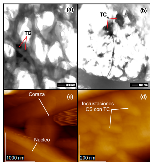
Figura 7. Microestructura de las fibras obtenidas por electrohilado de los polímeros de PCL/CS a una concentración w/w (8:1) disueltos en TFA/DCM a una concentración v/v (80:20) con una carga del 5 % w/w de TC respecto a 1 g de PCL (a,b) TEM y (c,d) AFM.
