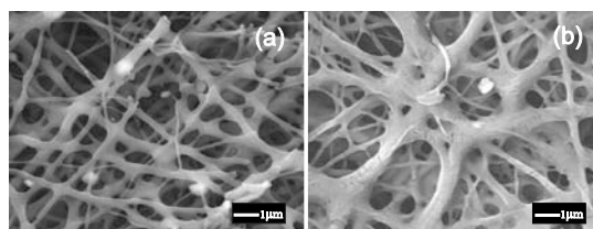
Figura 11. Micrografía SEM del estudio post-liberación de las membranas disueltas en PBS posterior a los 9 días: (a) PCL/CS w/w (8:1) y (b) PCL/CS w/w (10:1).
