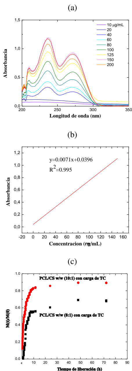
Figura 8. (a) Curvas de absorbancia de TC en solución buffer PBS al 0.1 M, (b) Curva de calibración empleada en los estudios de liberación de TC a \lambda = 235.56 nm y (c) Curvas de liberación de TC para las membranas de PCL/CS w/w (8:1) y (10:1), respectivamente.
