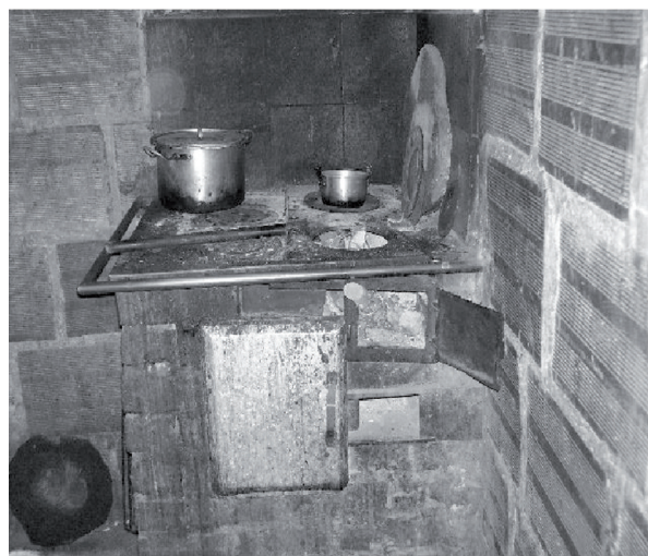
Figura 5b. Estufa tradicional tipo "caja".
