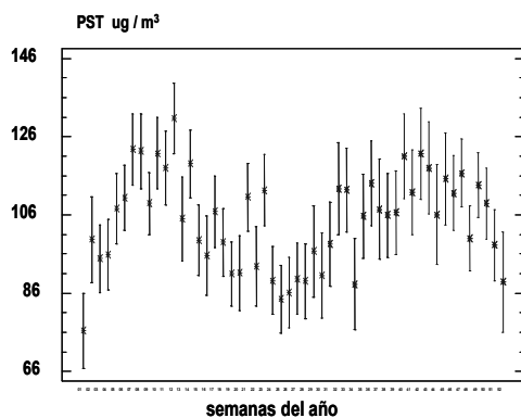
Figura 1. Comportamiento cíclico anual del material particulado en el aire. Medellín 2001-07
