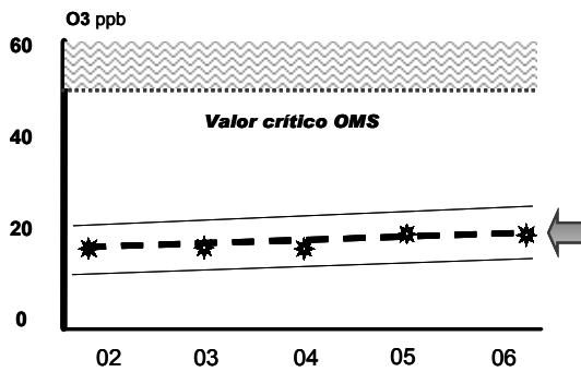
Figura 10. Niveles de Ozono (O 3 ). Promedios anuales, Medellín. 2001-07
