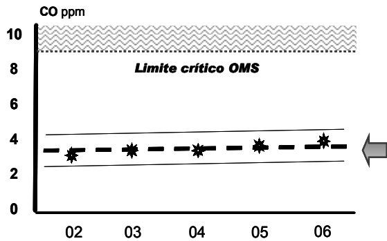
Figura 8. Niveles de Monóxido de Carbono (CO) Promedios anuales. Medellín 2001-07
