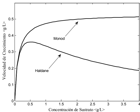
Figura 2. Modelos de crecimiento microbiano. Figure 2. Models for microbial growth
