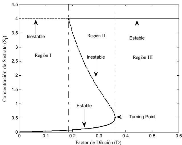
Figura 4. Diagrama de bifurcación del modelo de Haldane
