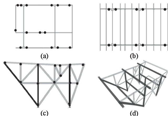
(a): planta de entrespiso, (b): planta de cubierta, (c): fachada lateral, (d): vista 3D
