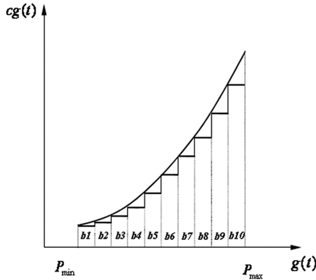
Figura 2. Aproximación por bloques de los costos de producción de una planta de generación
