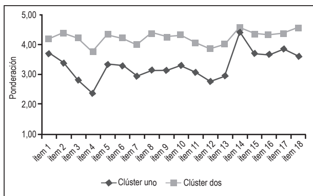
Gráfico 4. Análisis clúster
